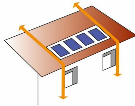
Implantation horizontale Alignement du champ de capteurs avec les ouvertures de façades
