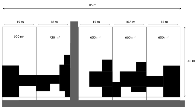
Parcellaire étroit et profond favorable à la cohérence du tissu urbain
