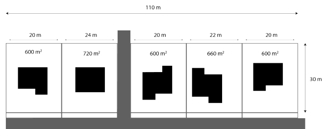
Linéaire de façade large peu structurant et coûteux pour la collectivité
