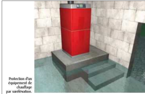
Mise hors d'eau d'un équipement de chauffage
