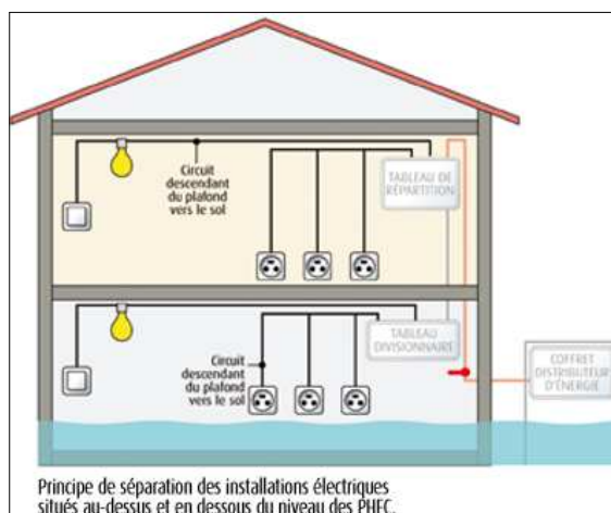
Réseau électrique descendant
