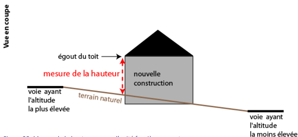
Figure 28: Mesure de la hauteur en cas d'unité foncière en pente
