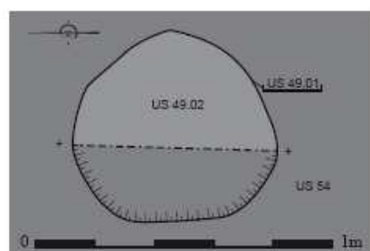
F 49 - Tr. 04 - plan et coupe nord/sud - 1/20
