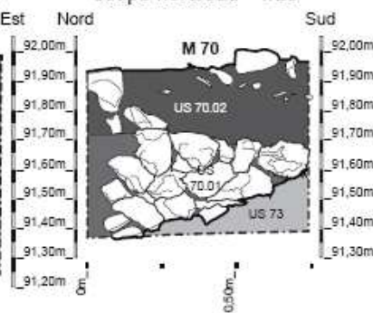
4) M 70 - Tr. 05 - coupe nord/sud - 1/20
