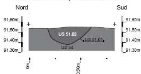
F 51 - Tr. 04 - coupe nord/sud - 1/20
