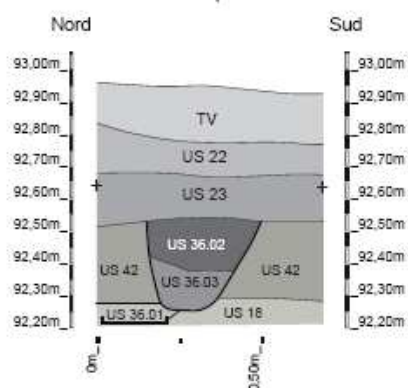
F 36 - Tr. 04 - coupe nord/sud - 1/20
