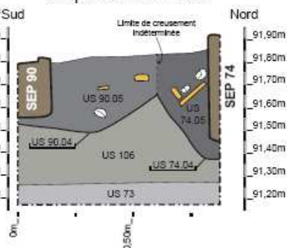
2) F 74 et 90 - Tr. 05 - Coupe sud/nord - 1/20
