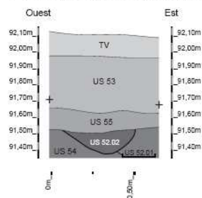
F 52 - Tr. 04 - coupe ouest/est - 1/20
