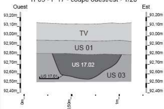
Tr 03 - F 17 - coupe ouest/est - 1/20
