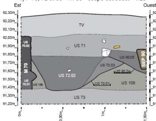
1) F 70, 72 et 90 - Tr. 05 - coupe est/ouest - 1/20
