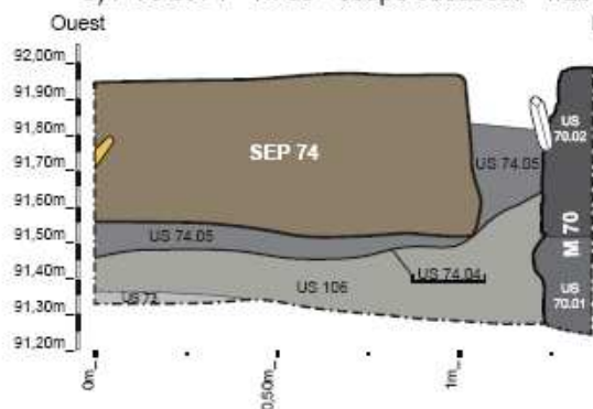
3) F 70 et 74 - Tr. 05 - coupe ouest/est - 1/20
