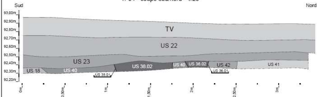
Tr 04 - coupe sud/nord - 1/20
