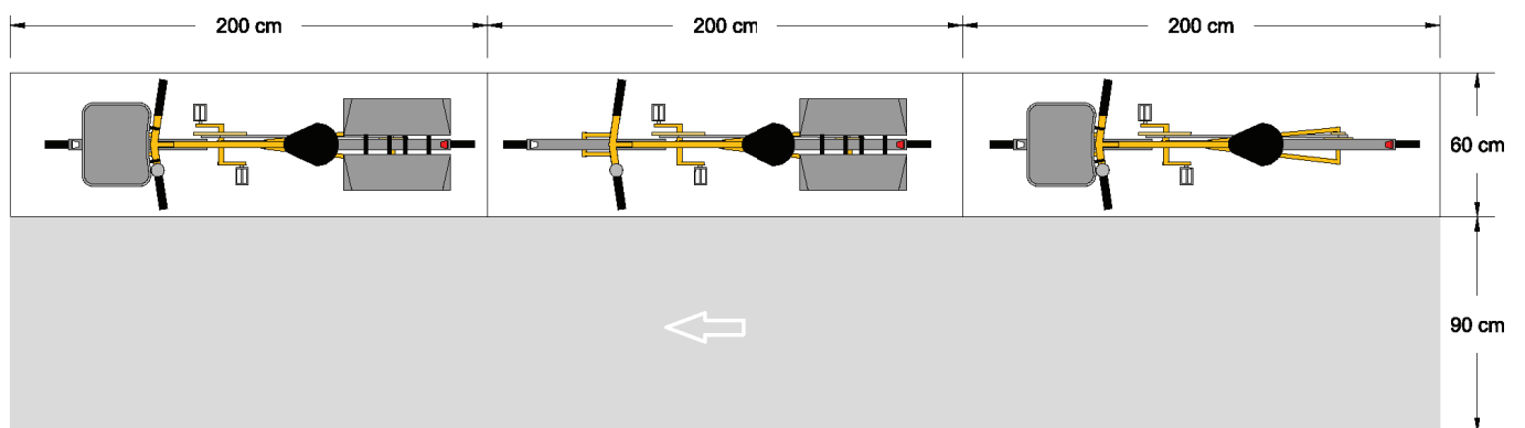
Figure 12 : Disposition longitudinale
