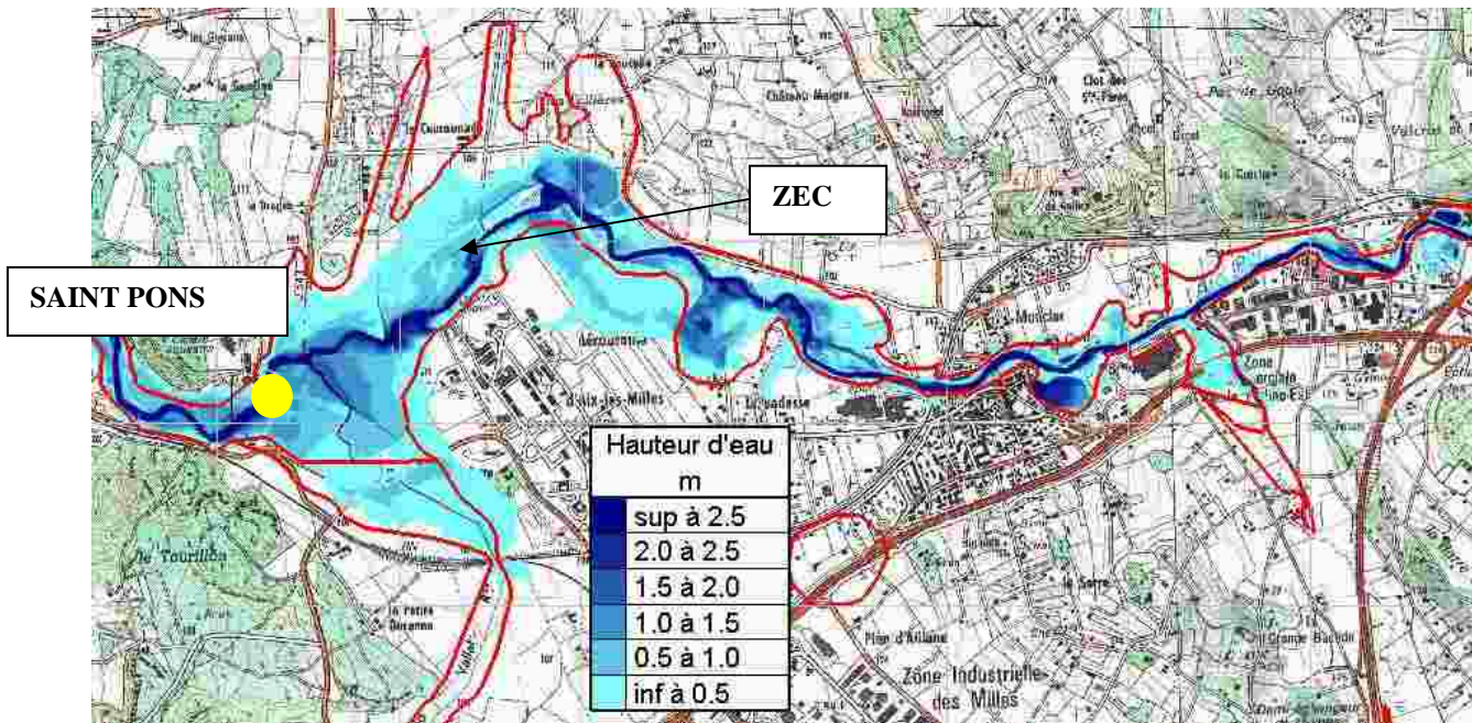
Figure 59 : Hauteur d'eau en 1978 dans la ZEC plaine des Milles
