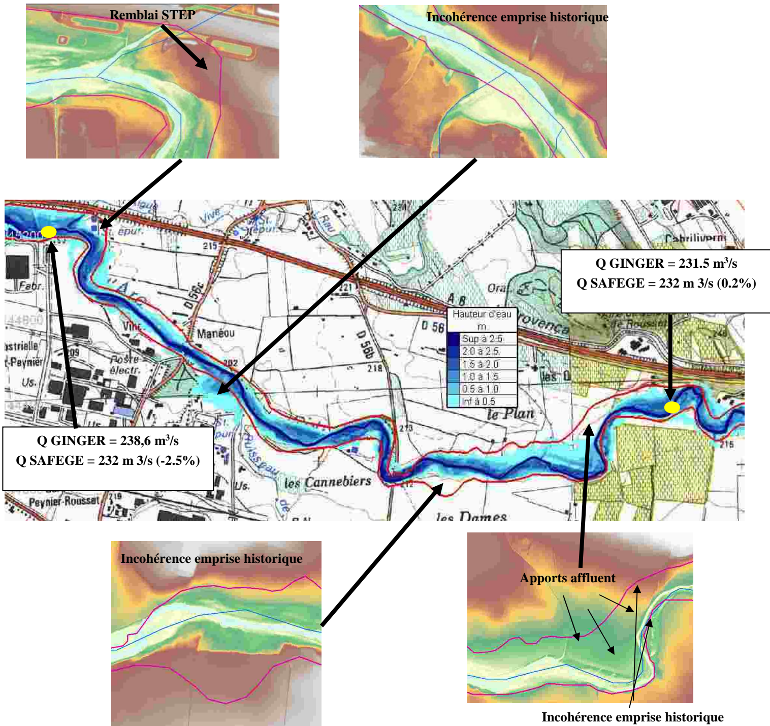
Figure 40 : zoom 1978 : amont de la zone industrielle de Rousset
