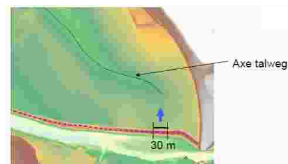
Figure 106 : Localisation de la rupture de la digue de Bachasson
