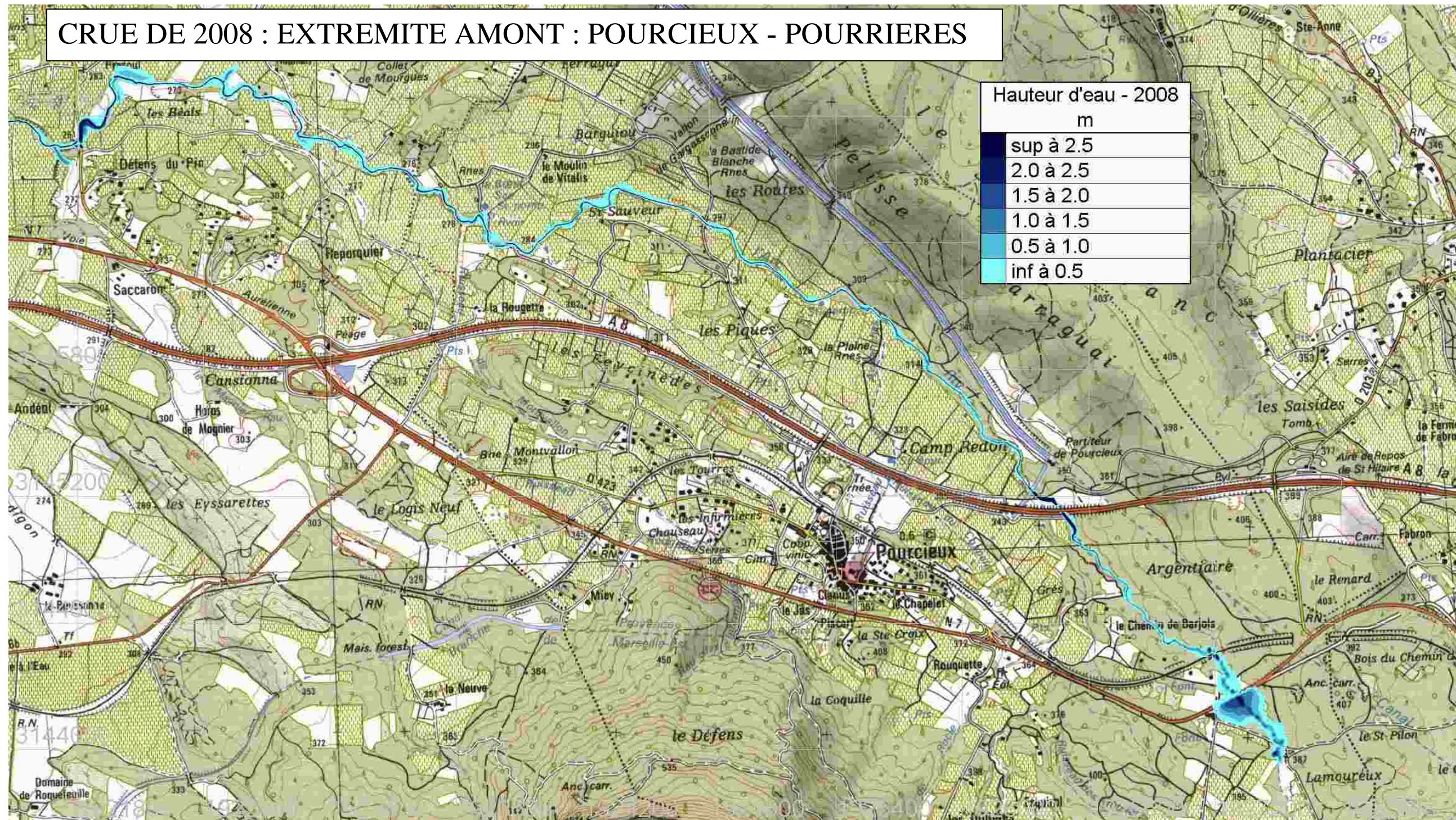
Figure 64 : Cartes des hauteurs d'eau pour la crue de 2008 –modèle amont
