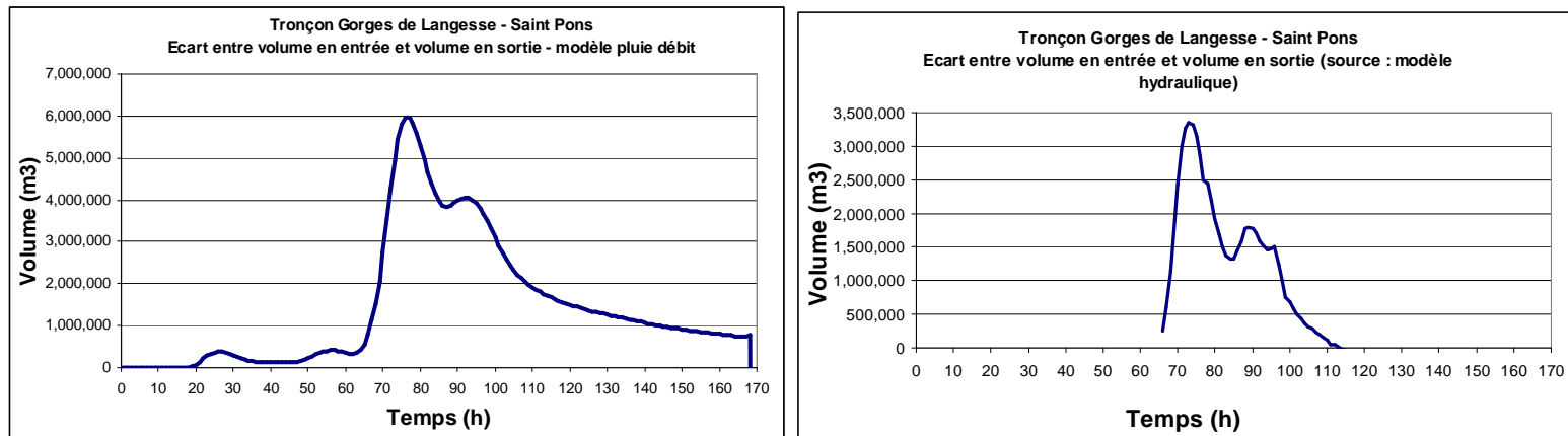
Figure 62 : Écart au cours du temps entre le volume en entrée et le volume en sortie sur le tronçon Gorges de Langesse/ Saint Pons pour le modèle pluie débit et le modèle hydraulique
