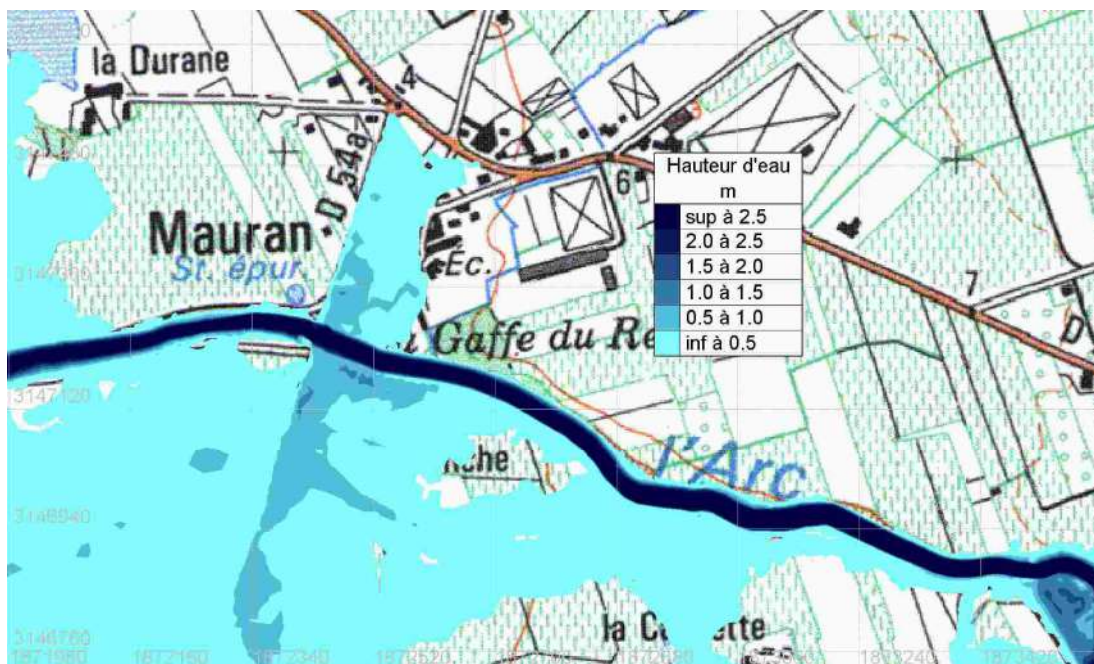
Figure 78 : Crue de 2008 au hameau de Mauran (Berre)
