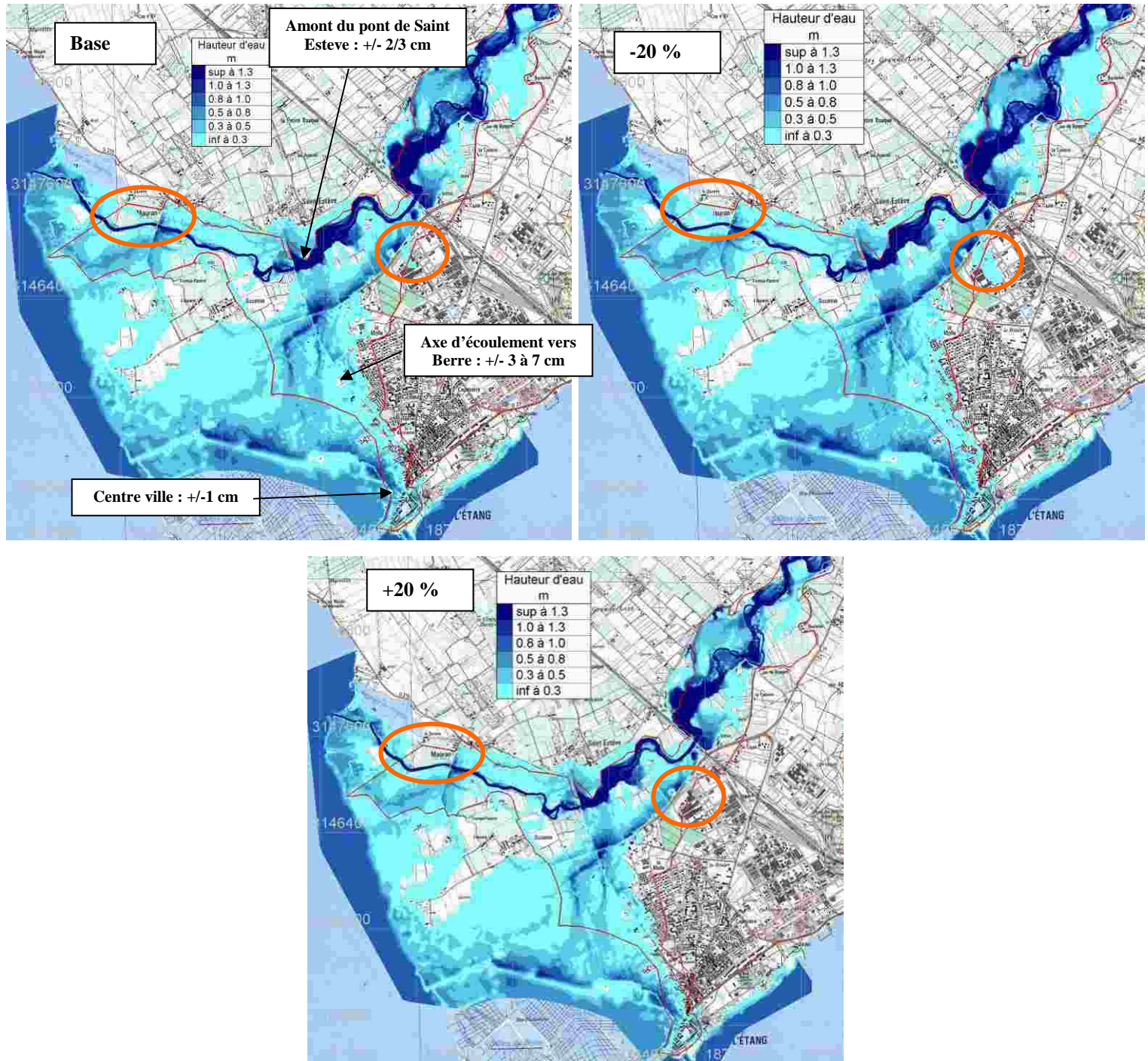
Figure 85 : Comparaison modèle de base – modèle Strickler +/- 20% - Plaine de Berre l'étang
