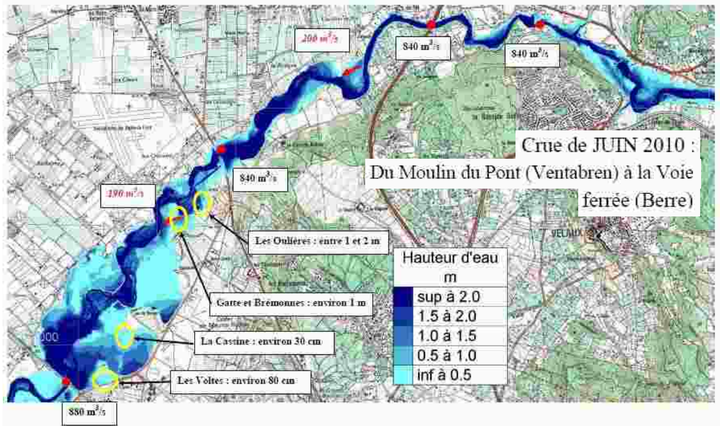
Figure 103 : hauteurs d'eau de référence (entre le Moulin du Pont et la voie ferrée de Berre)
