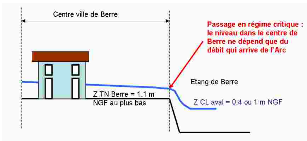
Figure 88 : Schéma de principe de la ligne d'eau dans le centre-ville de Berre
