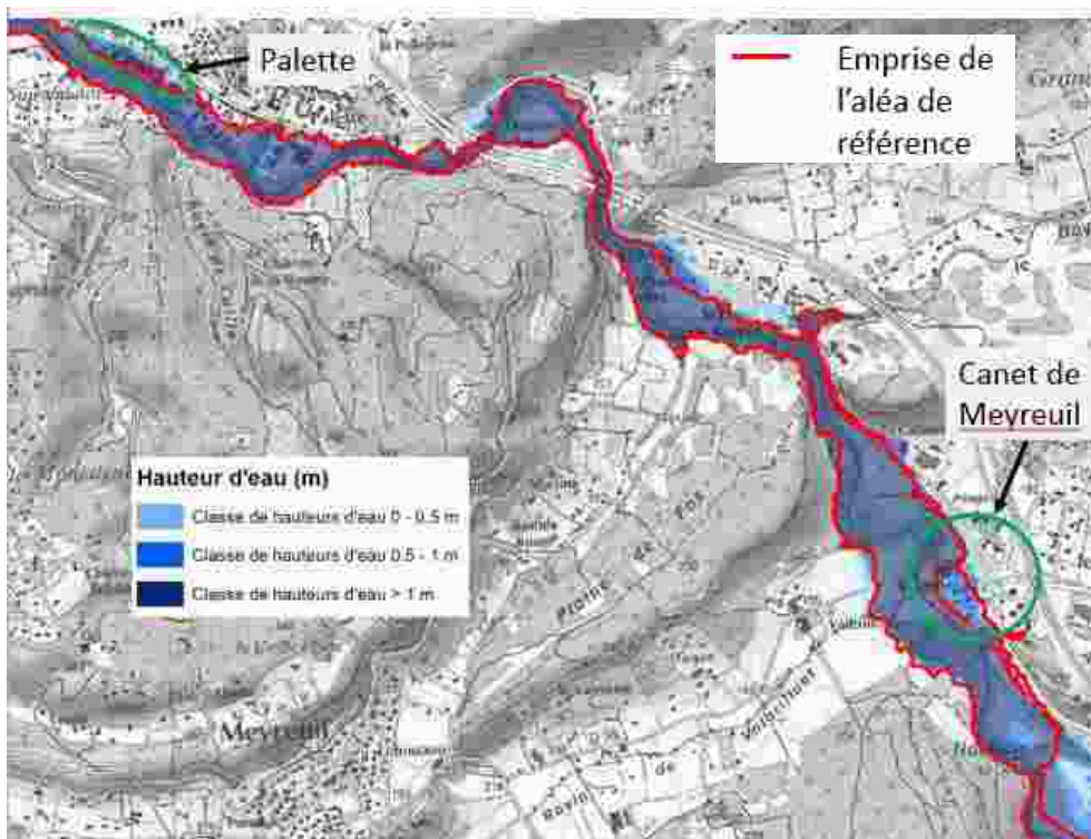
Figure 109 : Hauteurs de la crue exceptionnelle – secteur de Meyreuil – Le Tholonet
