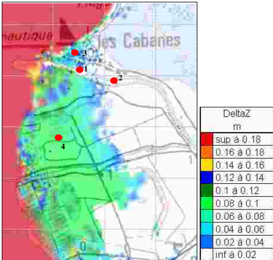
Figure 86 : Impact du choix de la condition limite aval sur les niveaux d'eau (secteur de la confluence de l'Arc avec l'étang de Berre)
