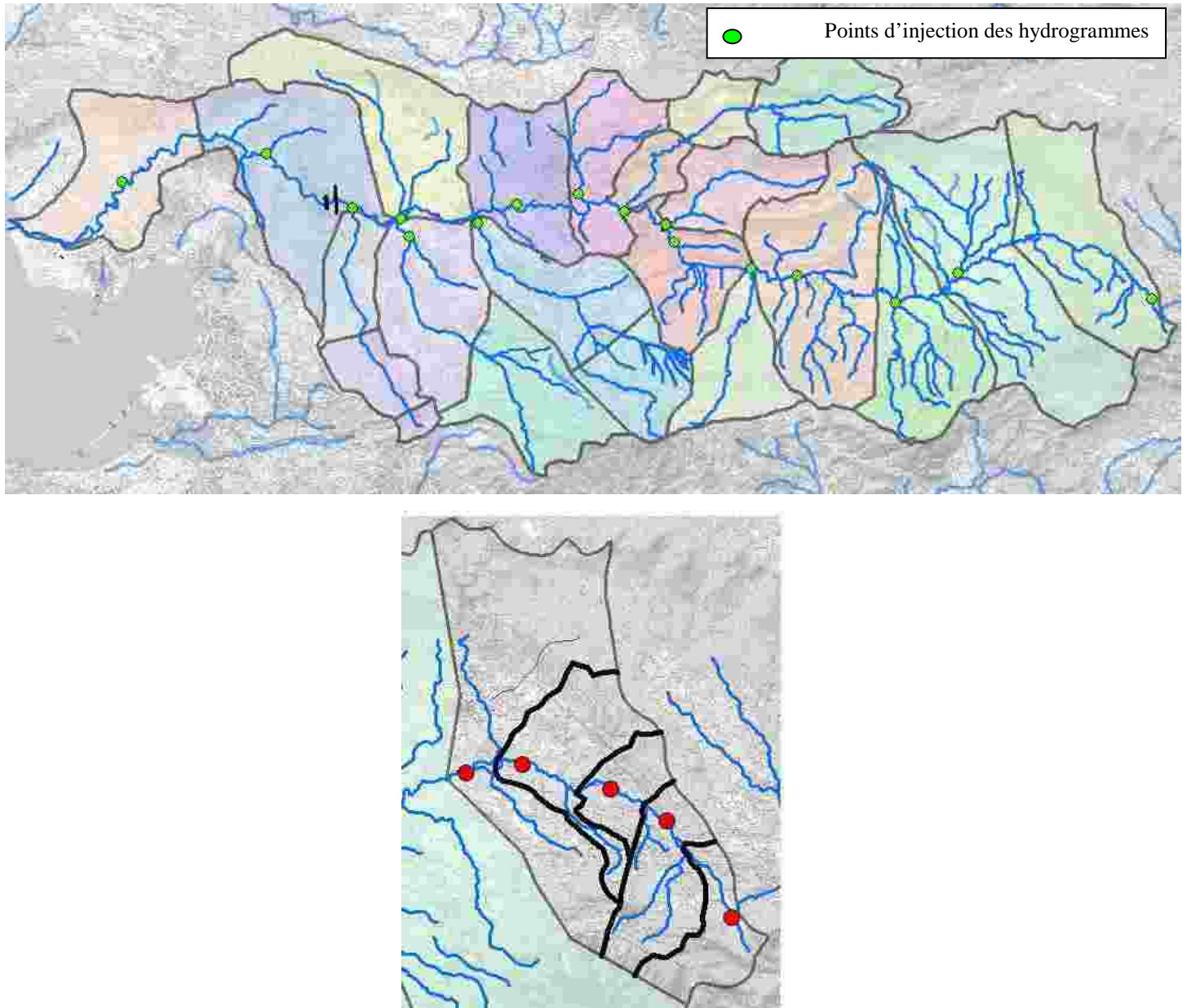
Figure 25 : Localisation des points d'injection des hydrogrammes
