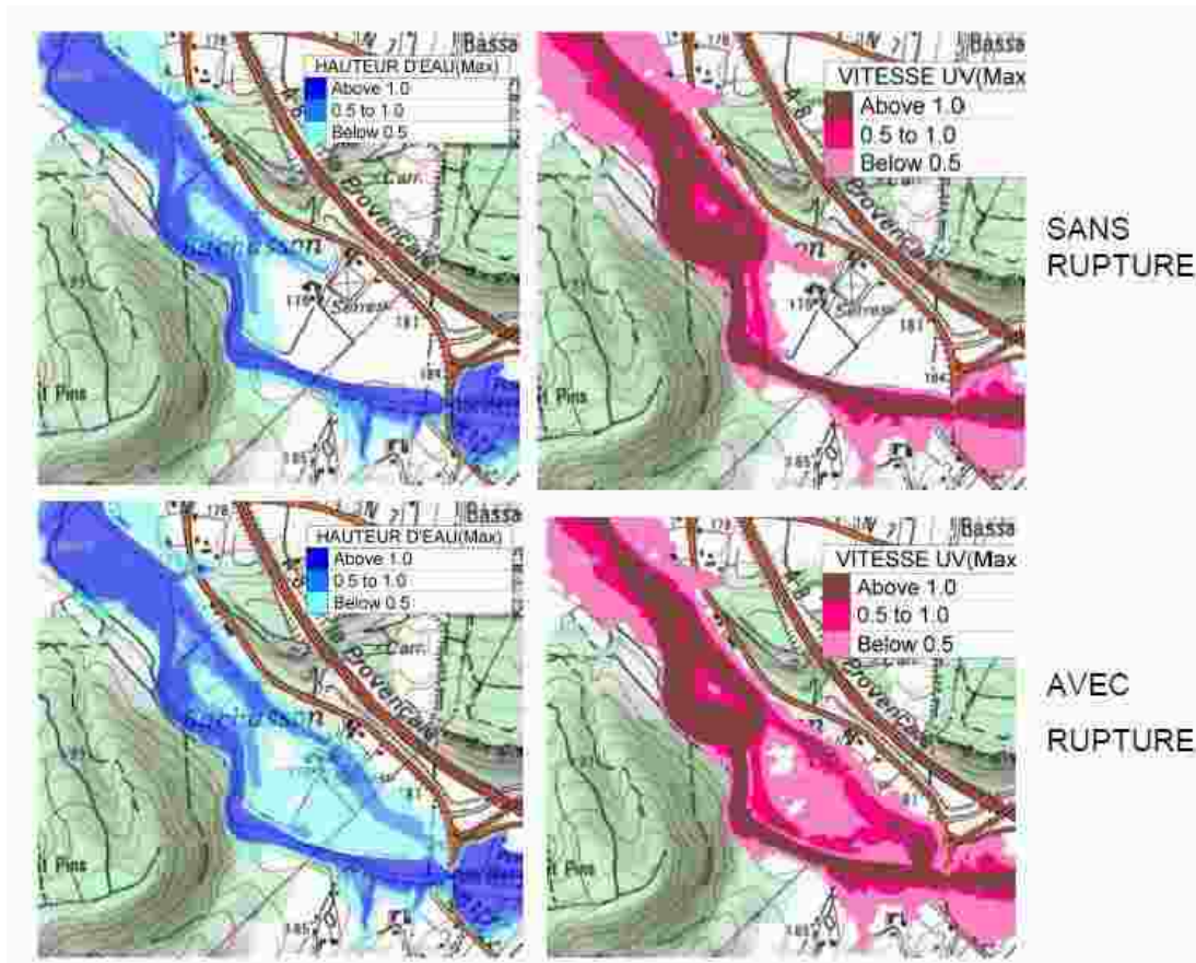
Figure 107 : Impact de la rupture de la digue de Bachasson
