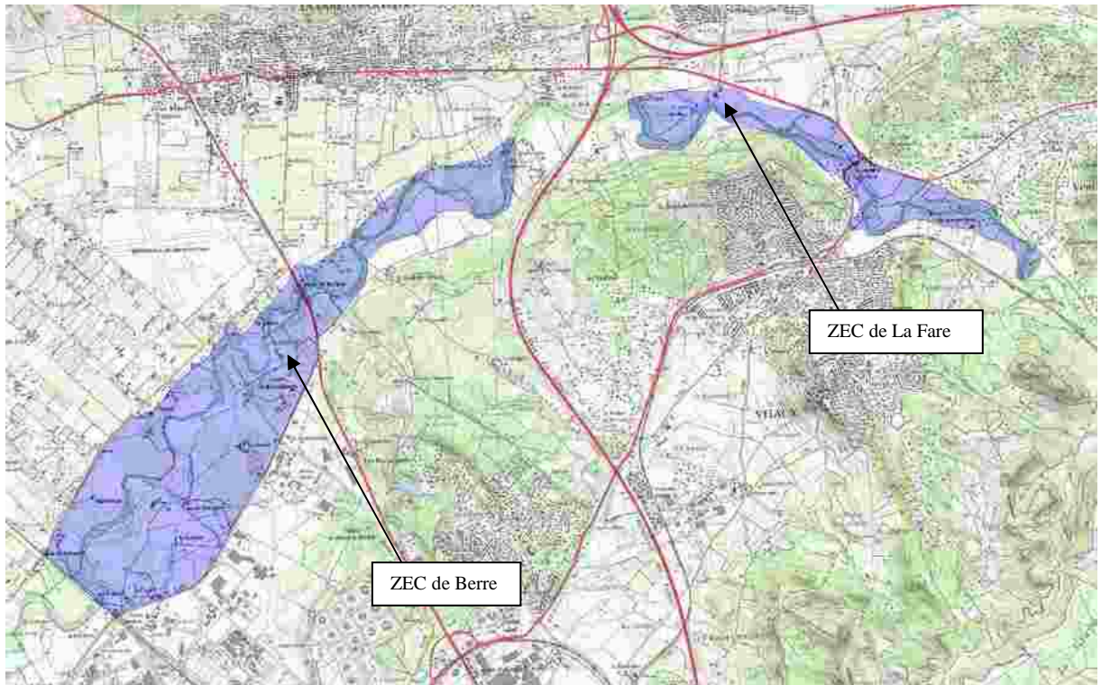
Figure 4 : Fonctionnement hydraulique de l'Arc – en aval des gorges de Roquefavour
