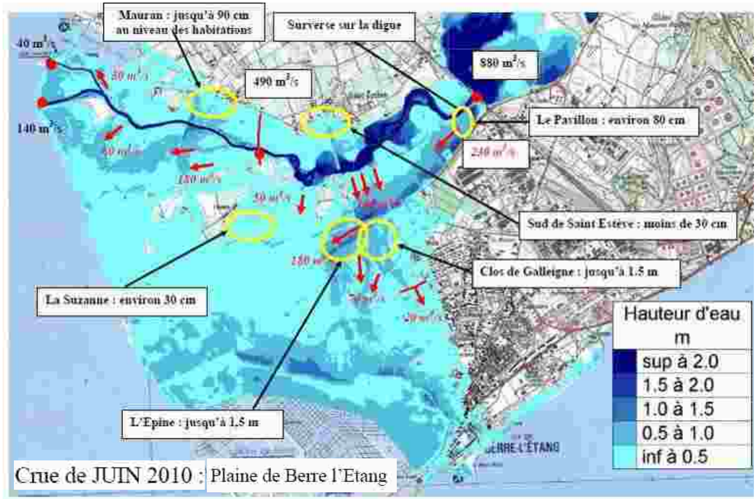
Figure 104 : hauteurs d'eau de référence (Plaine de Berre l'Étang)
