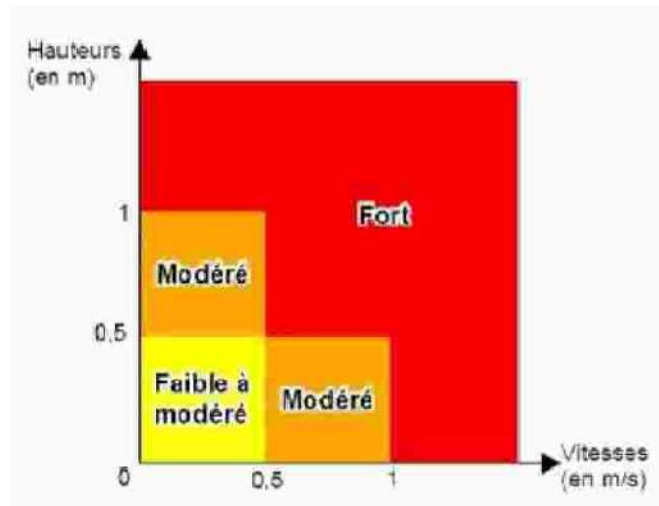
Figure 105 : grille d'aléa
