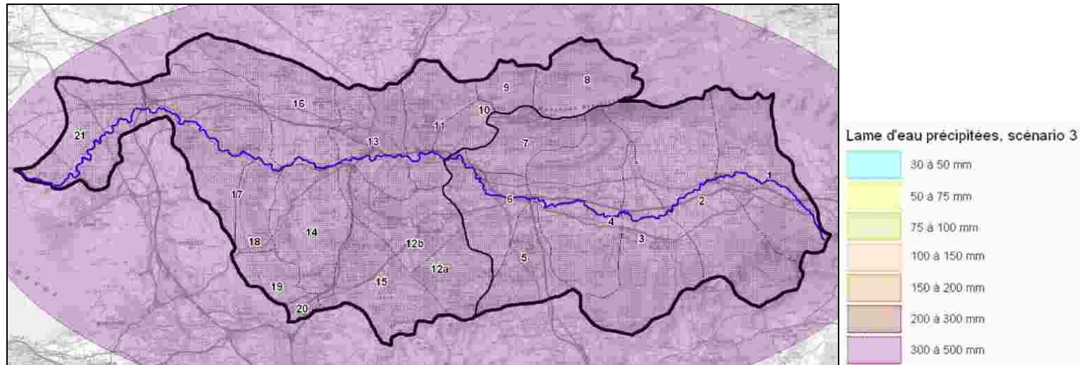
Figure 13 : Lame d'eau précipitée pour les 3 scénarii – Extrait de « L'Évaluation de l'incidence hydrologique sur le bassin versant de l'Arc d'un épisode pluvieux tel que celui qui a affecté le var le 15 juin 2010 – GINGER – SABA – 2010 »
