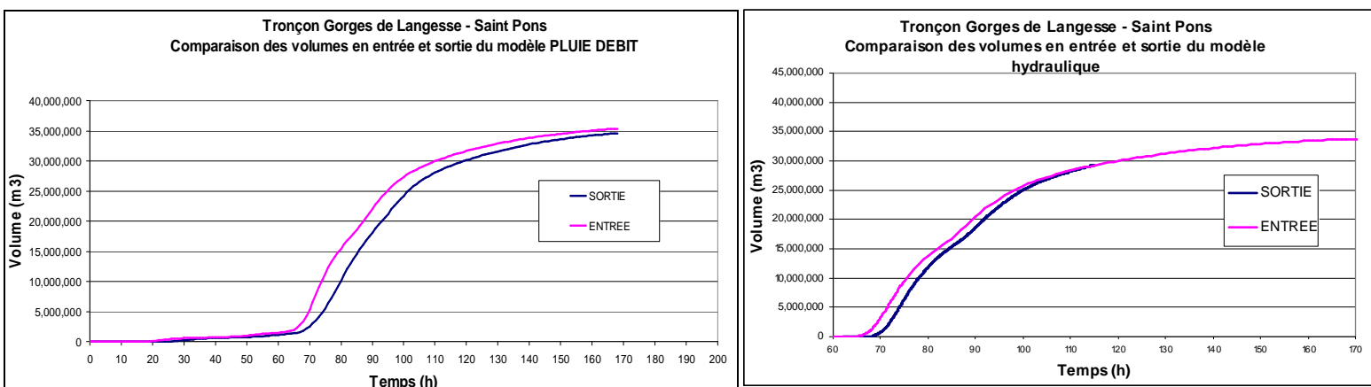
Figure 61 : Volumes cumulés pour la crue de 1978 pour le modèle pluie-débit et le modèle hydraulique – tronçon Gorges de Langesse/ Saint Pons
