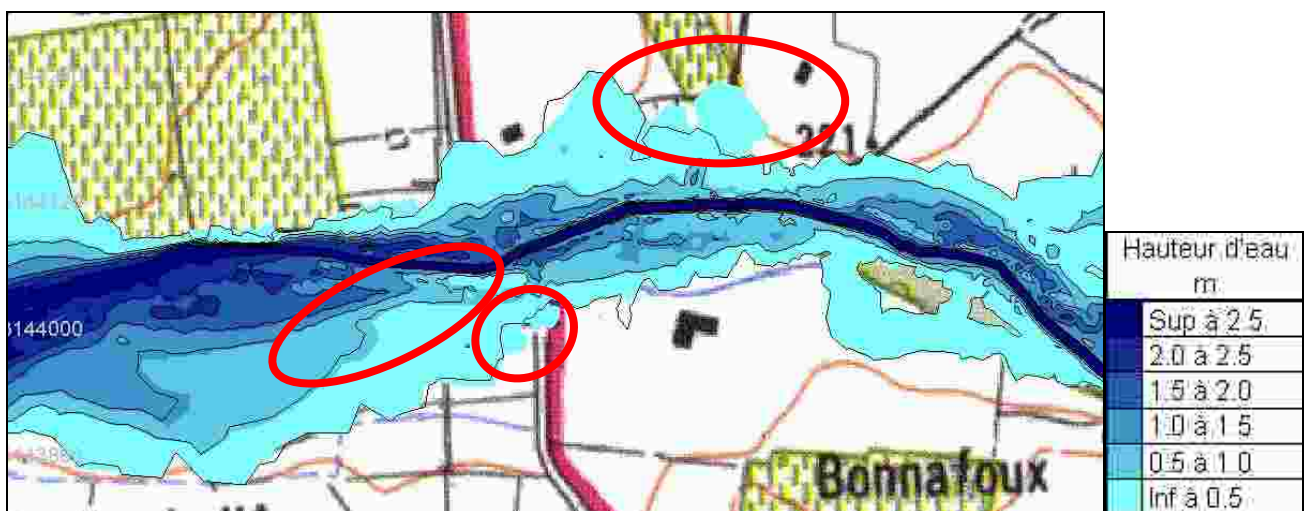
Figure 81 : Comparaison modèle de base – modèle Strickler +20%
