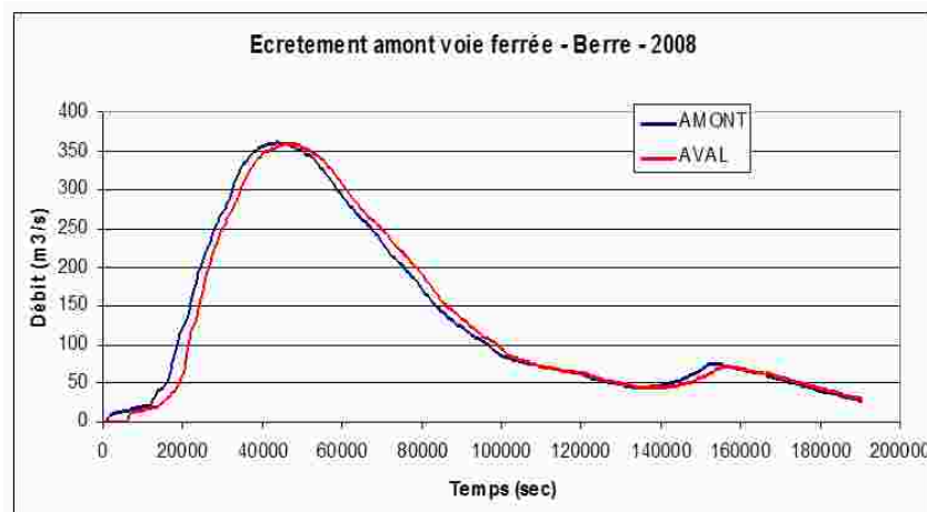
Figure 11 : Hydrogrammes de la crue de 2008 en amont de la voie ferrée de Berre
