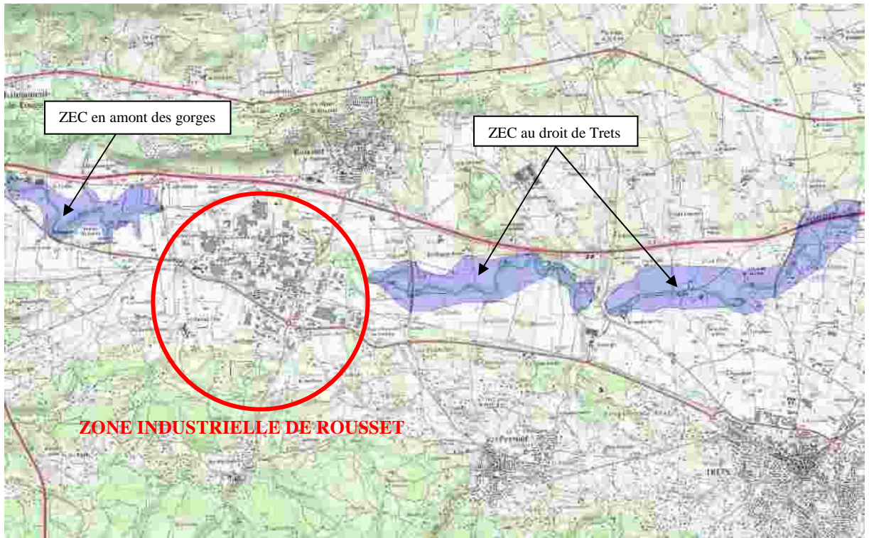
Figure 2 : Fonctionnement hydraulique de l'Arc : de Trets aux gorges de Langesse
