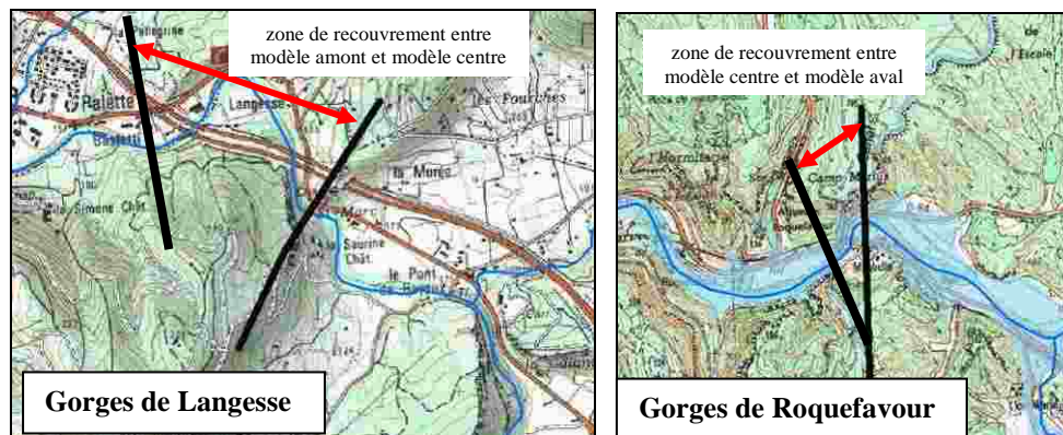
Figure 23 : zone de recouvrement des modèles hydrauliques
