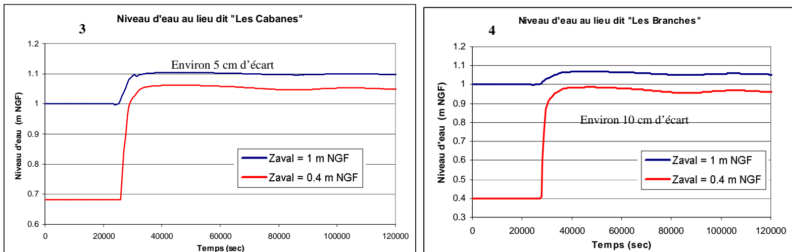
Figure 87 : Courbes des niveaux d'eau en fonction du temps à proximité de la confluence Arc/Etang de Berre pour les deux conditions limite aval testées
