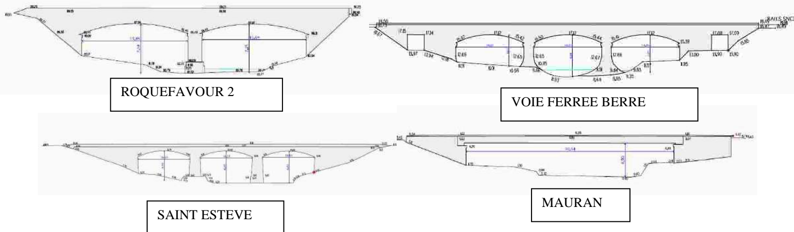
Figure 37 : Coupes des ouvrages à débitance limitée
