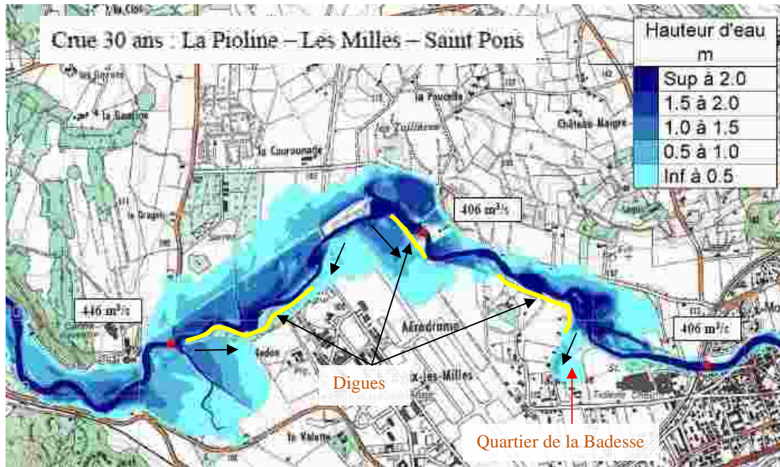
Figure 94 : Hauteurs de la crue trentennale – secteur La Pioline – Les Milles – Saint Pons
