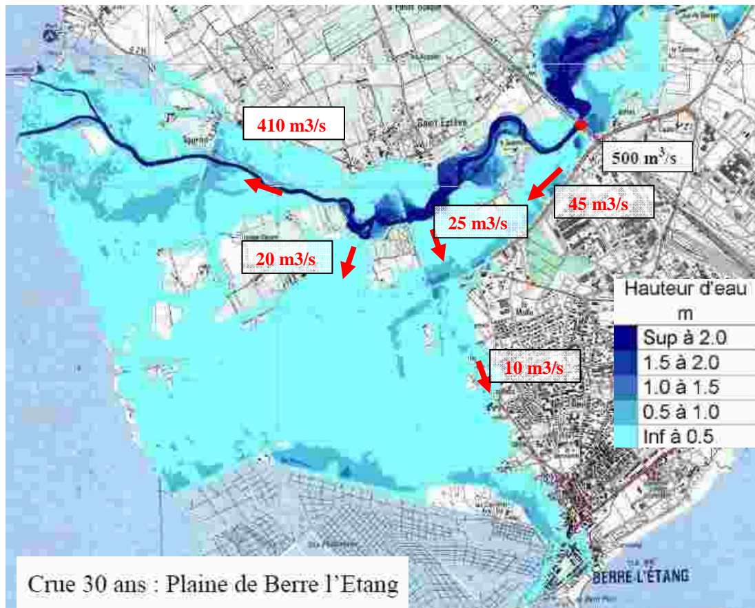
Figure 96 : Hauteurs de la crue trentennale – plaine de Berre l'Étang
