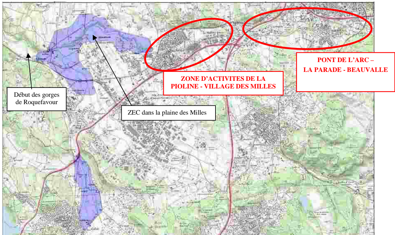
Figure 3 : Fonctionnement hydraulique de l'Arc- secteur d'Aix en Provence
