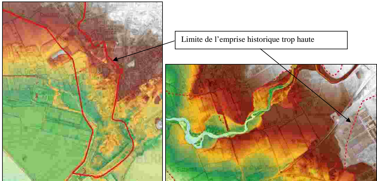
Figure 51 : comparaison LIDAR et emprise historique de 1978 à Berre l'Étang
