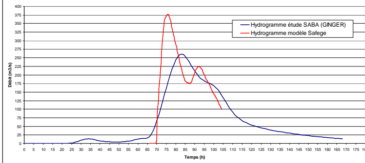
Comparaison des données du modèle pluie débit avec le modèle hydraulique - au niveau de l'A7 à Berre
