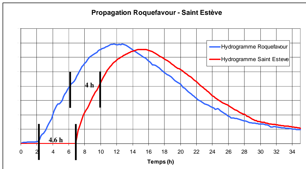
Figure 79 : Propagation des hydrogrammes d'après le modèle hydraulique
