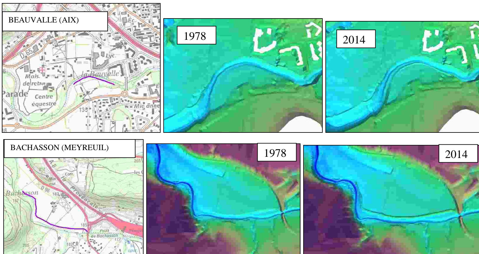
Figure 33 : Localisation des modifications apportées au maillage pour modélisation de la crue de 1978
