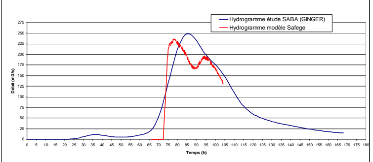
Comparaison des données du modèle pluie débit avec le modèle hydraulique - au niveau de Mauran (BERRE)
