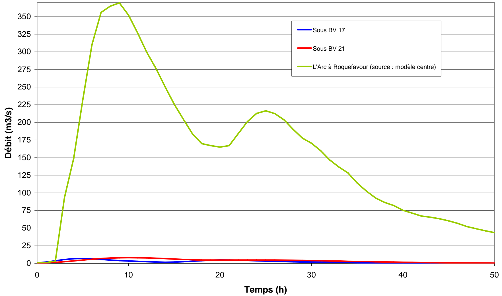
Crue de 1978 - Hydrogrammes injectés dans le modèle aval
