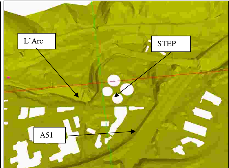
Vue lidar du MNT (modèle numérique de terrain) : 1 point tous les mètres –relevé par avion
