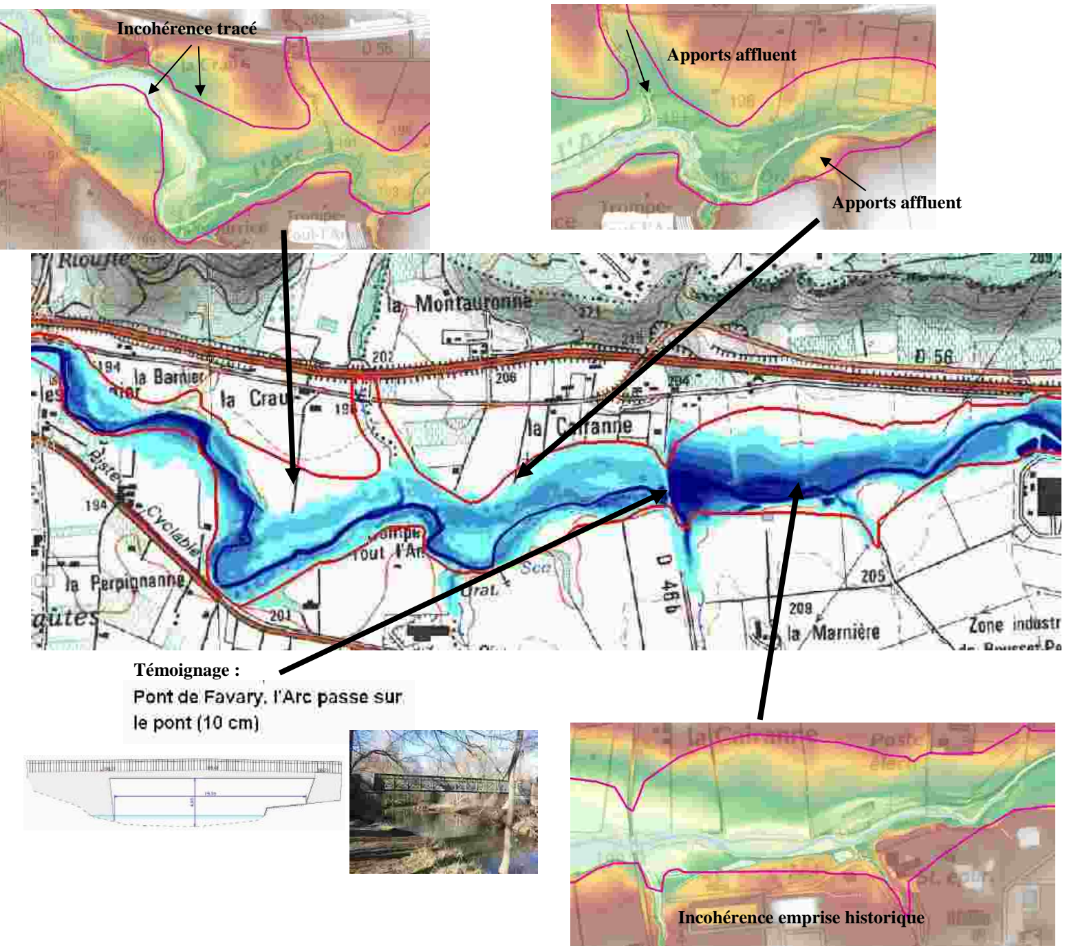
Figure 41 : zoom 1978 : secteur de Favary (Rousset)
