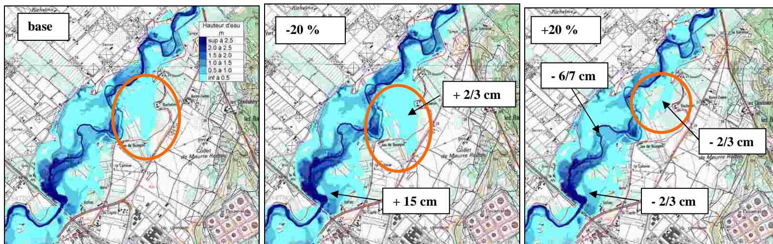
Figure 84 : Comparaison modèle de base – modèle Strickler +/- 20% - Amont de la voie ferrée à Berre l'étang
