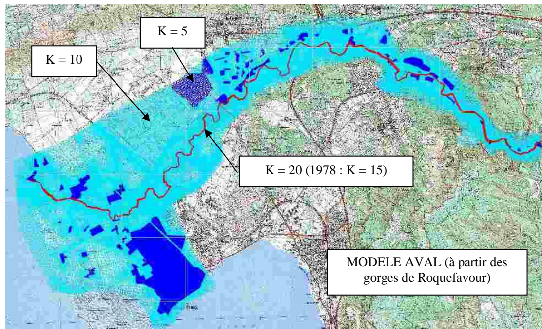
Figure 36 : localisation des différentes rugosités appliquées dans le modèle hydraulique
