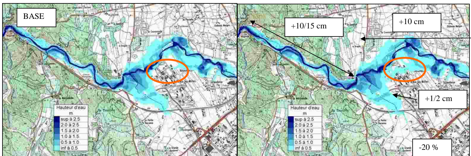
Figure 83 : Comparaison modèle de base – modèle Strickler -20% - ZEC plaine des Milles
