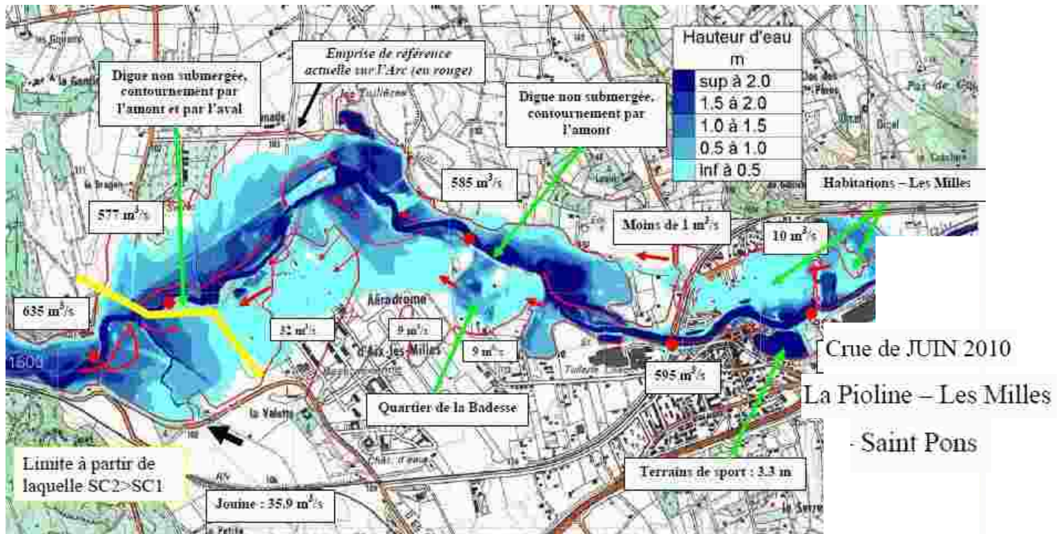
Figure 100 : hauteurs d'eau de référence (La Pioline, Les Milles, Saint Pons)
