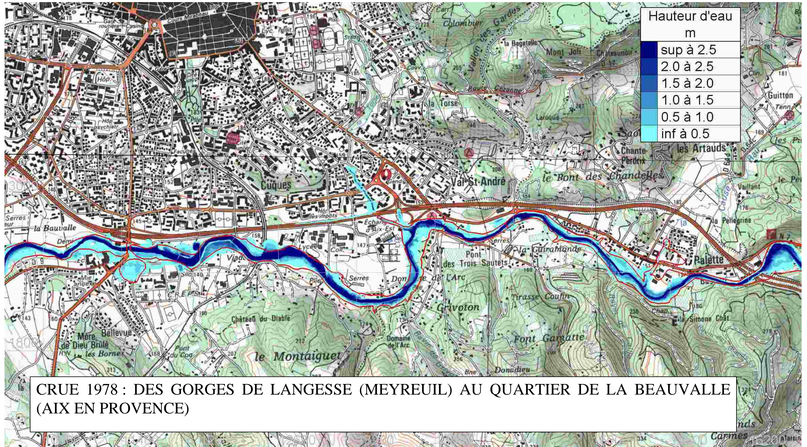
Figure 44 : Cartes de hauteurs et vitesses maximale pour la crue de 1978 (secteur des gorges de Langesse aux gorges de Roquefavour)
