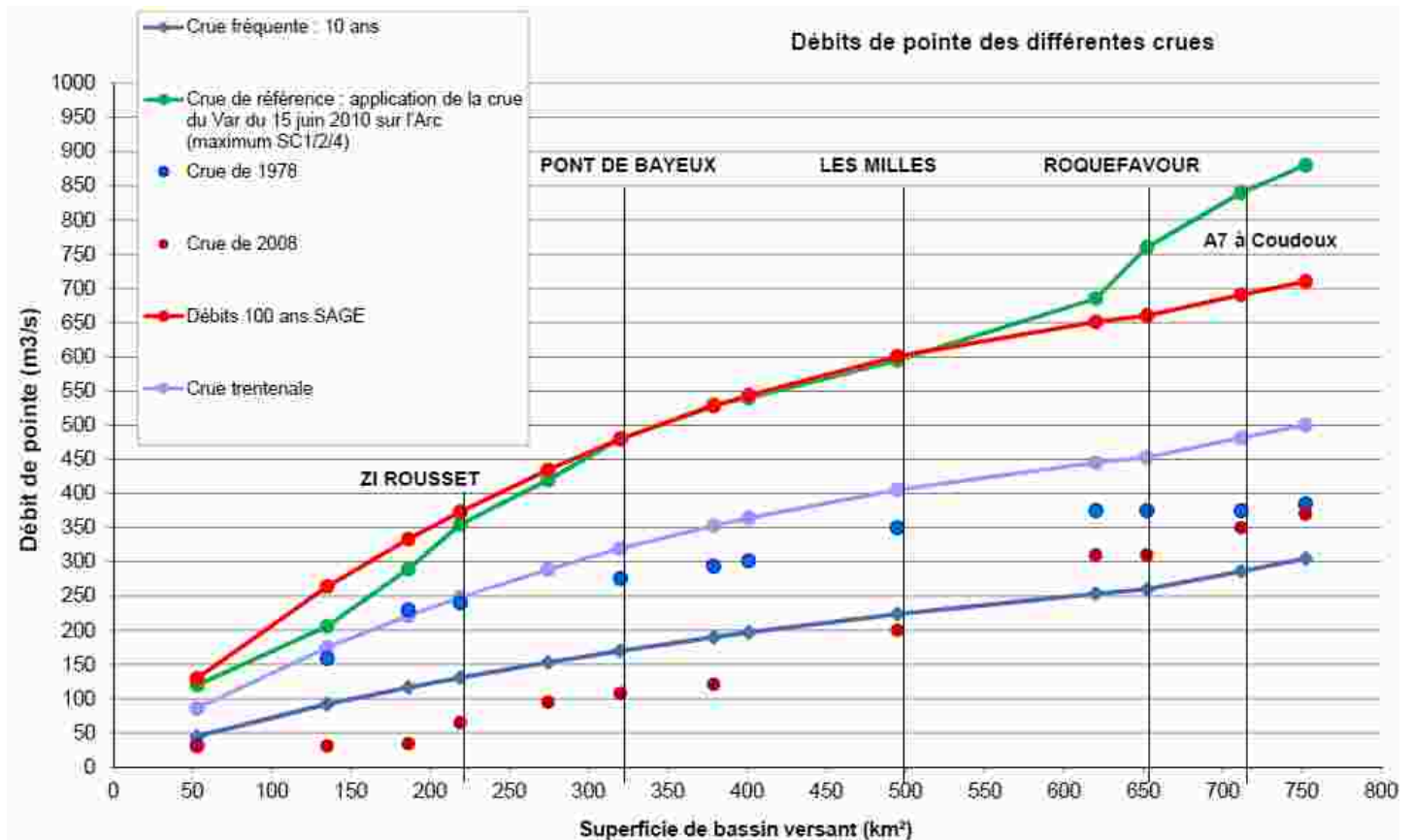
Figure 19 : Graphique des débits retenus pour le TRI de l'Arc
