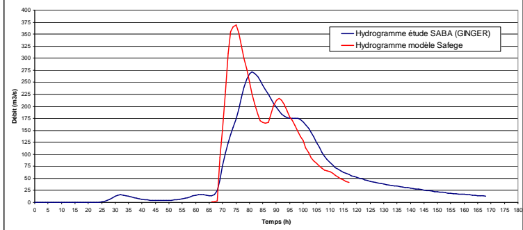
Comparaison des données du modèle pluie débit avec le modèle hydraulique - ROQUEFAVOUR
