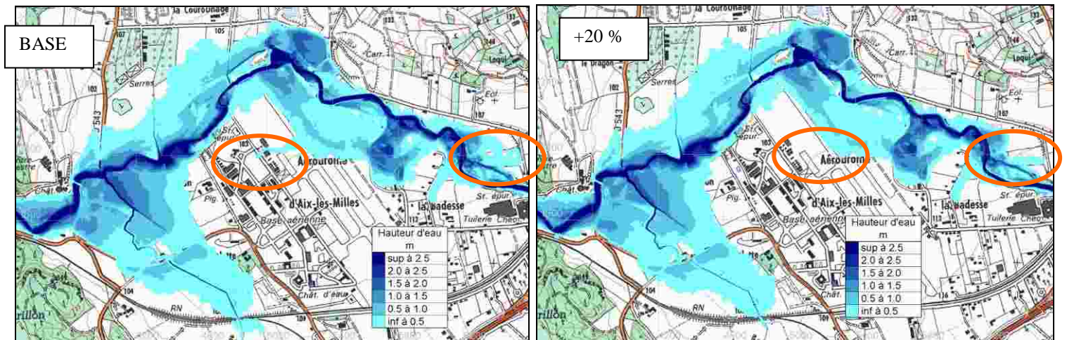
Figure 82 : Comparaison modèle de base – modèle Strickler +20% - plaine des Milles
