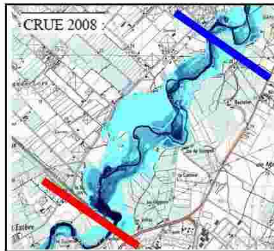
Figure 10 : Inondation de 2008 en amont de la Voie ferrée de Berre
