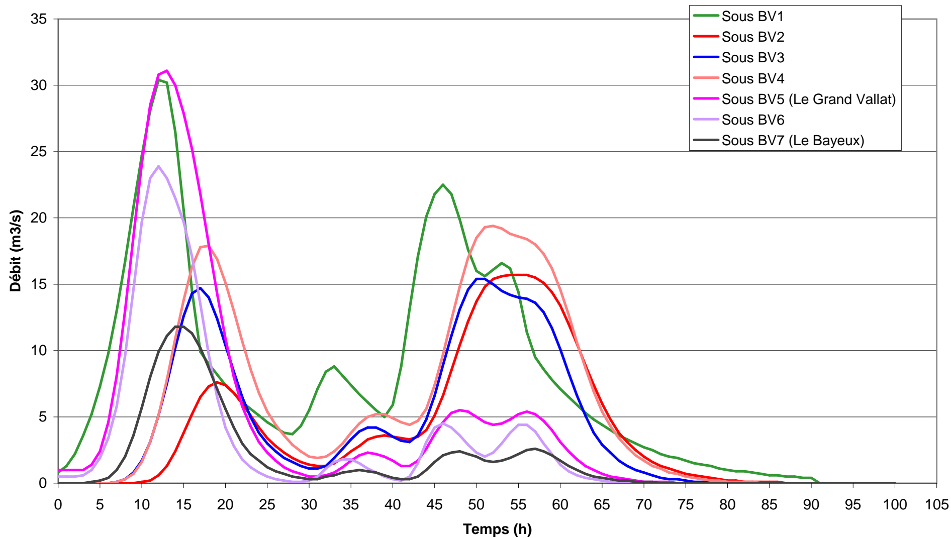
Crue de 2008 - hydrogrammes injectés dans le modèle amont
