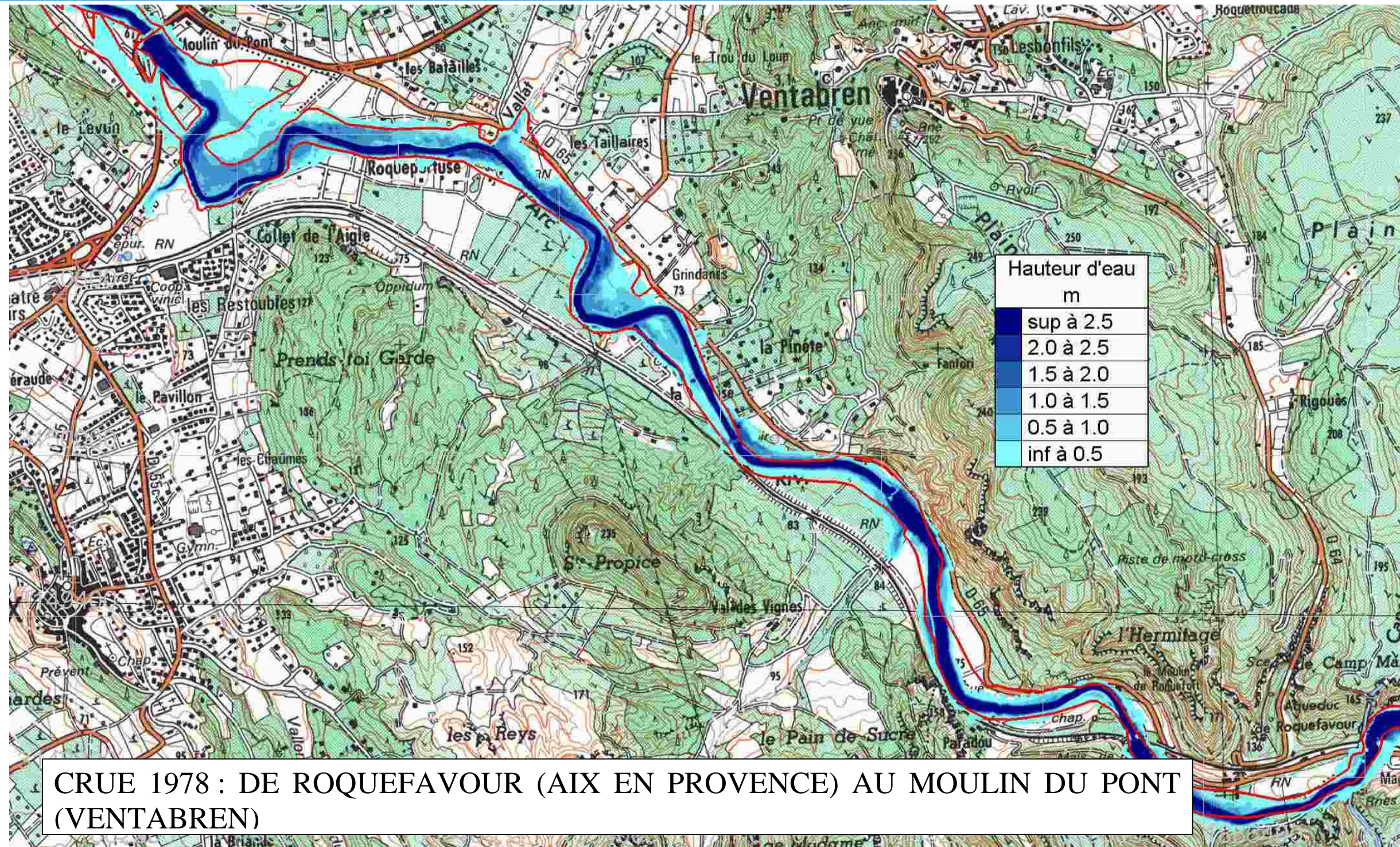
Figure 48 : Cartes des hauteurs et vitesses maximales pour la crue de 1978 – secteur Gorges de Roquefavour / Étang de Berre
