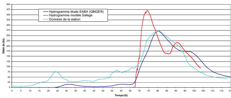
Comparaison des données du modèle pluie débit avec le modèle hydraulique - au niveau de l'A7 à Berre
