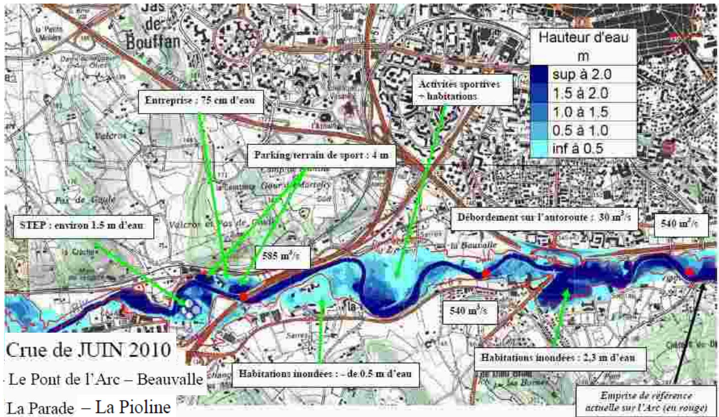
Figure 99 : hauteurs d'eau de référence (Pont de l'Arc, Beauvalle, La Parade, La Pioline)
