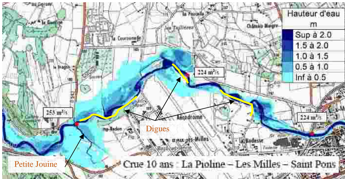
Figure 90 : hauteurs d'eau décennales (La Pioline, Les Milles, Saint Pons)
