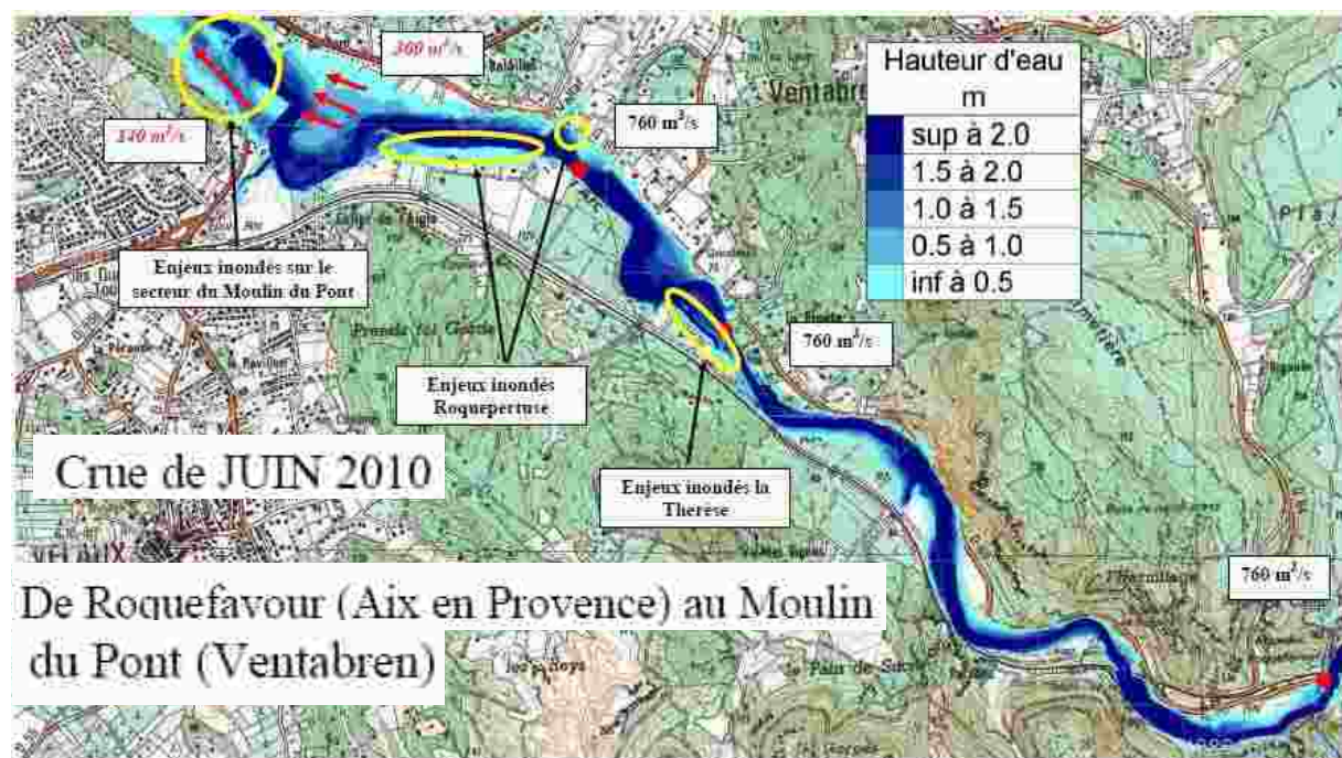
Figure 102 : hauteurs d'eau de référence (entre la ZEC des Milles et Roquefavour)
