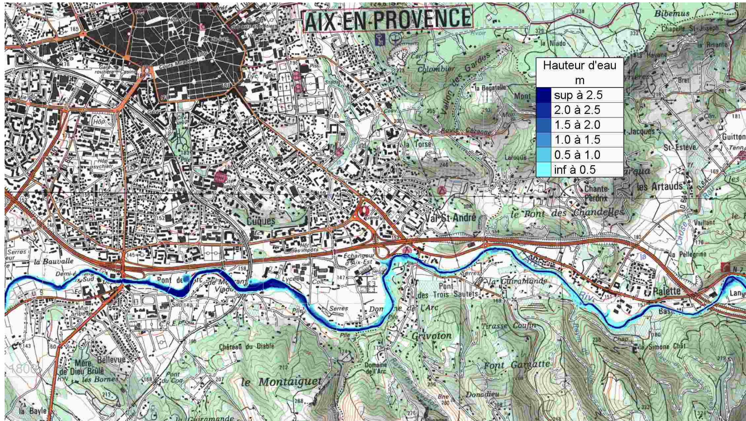
Figure 65 : Cartes des hauteurs d'eau pour la crue de 2008 – modèle centre
