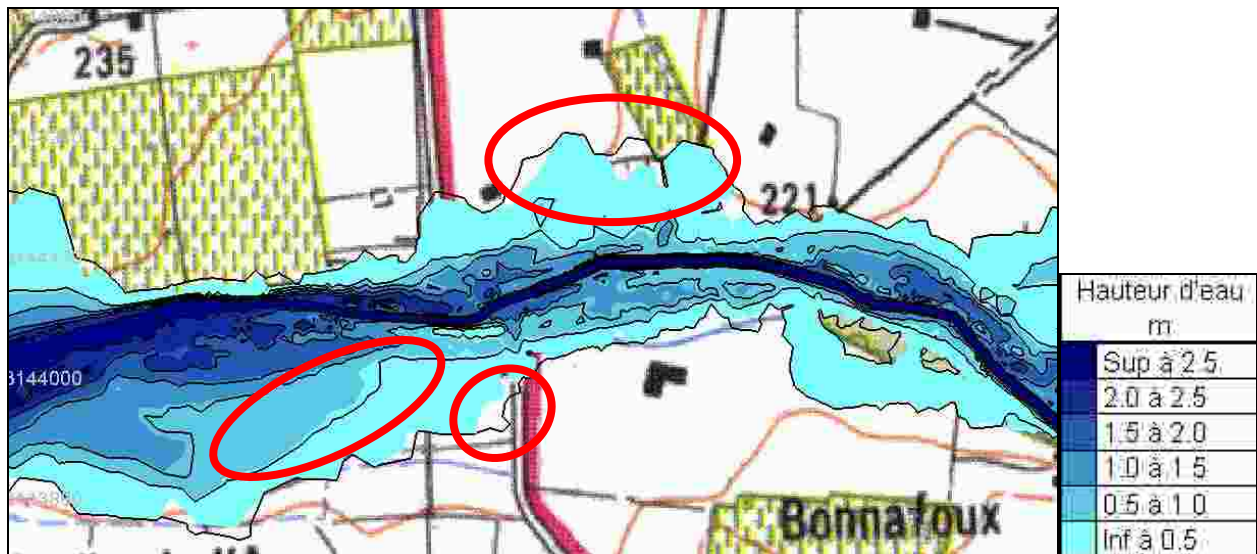
Figure 80 : Comparaison modèle de base – modèle Strickler -20%
