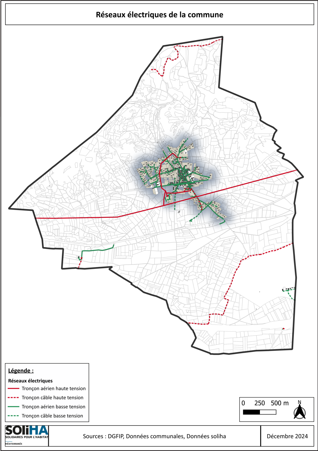
Réseaux électrique de la commune
