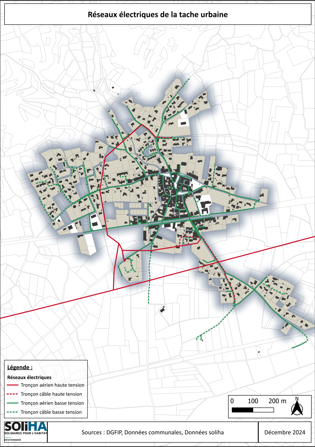
Réseaux électriques de la tache urbaine
