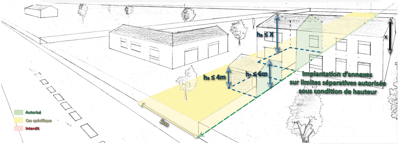
Schéma 36 : Hauteur des constructions, cas particulier (Article A10, Paragraphe 3) :
