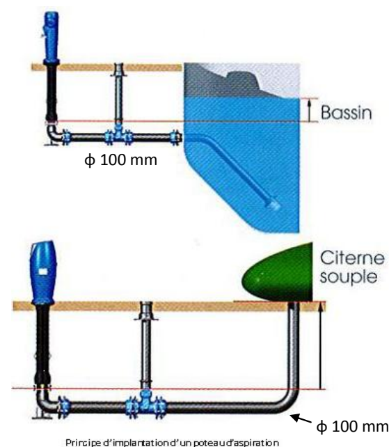
Principe d'implantation d'un poteau d'aspiration
