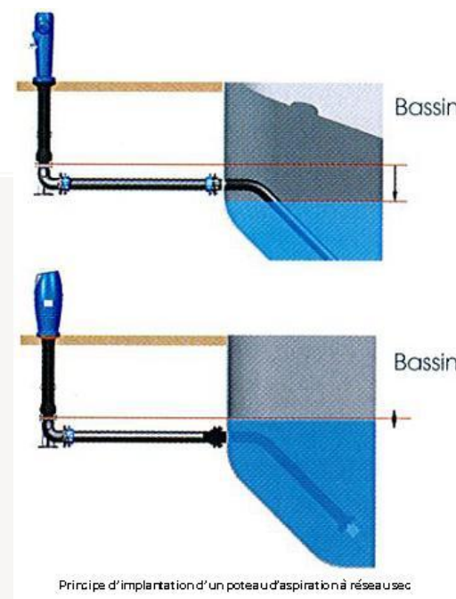
Principe d'implantation d'un poteau d'aspiration à réseau sec
