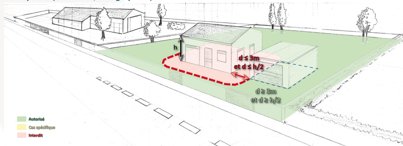
Schéma 39 : Implantation des constructions les unes par rapport aux autres sur une même propriété (Article N8, Paragraphe 1) :
