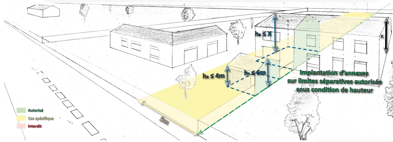
Schéma 40 : Hauteur des constructions, cas particulier (Article N10, Paragraphe 3) :
