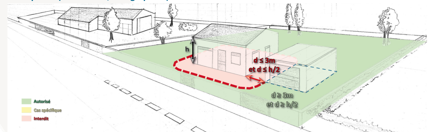
Schéma 24 : Hauteur des constructions, cas particulier (Article AU10, Paragraphe 3) :
