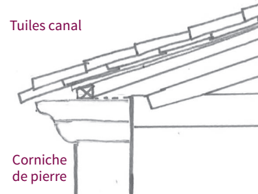
Coupe départ de toiture : corbeau en pierre, saillant du mur qui soutient le départ de toit à chaque extrémité
