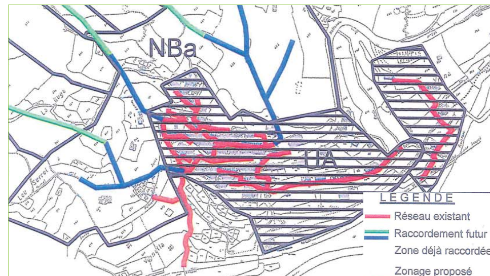
SCHÉMA D'ASSAINISSEMENT DE TOUËT-DE L'ESCARÈNE
