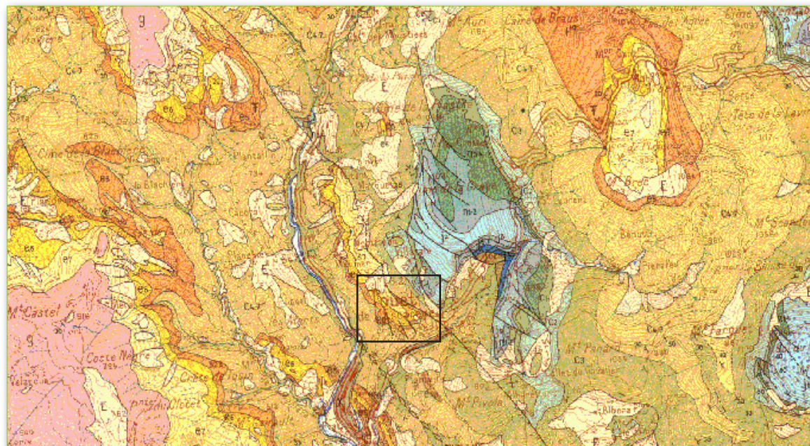
LA GÉOLOGIE SUR LE TERRITOIRE COMMUNAL DE TOUËT-DE-L'ESCARÈNE
