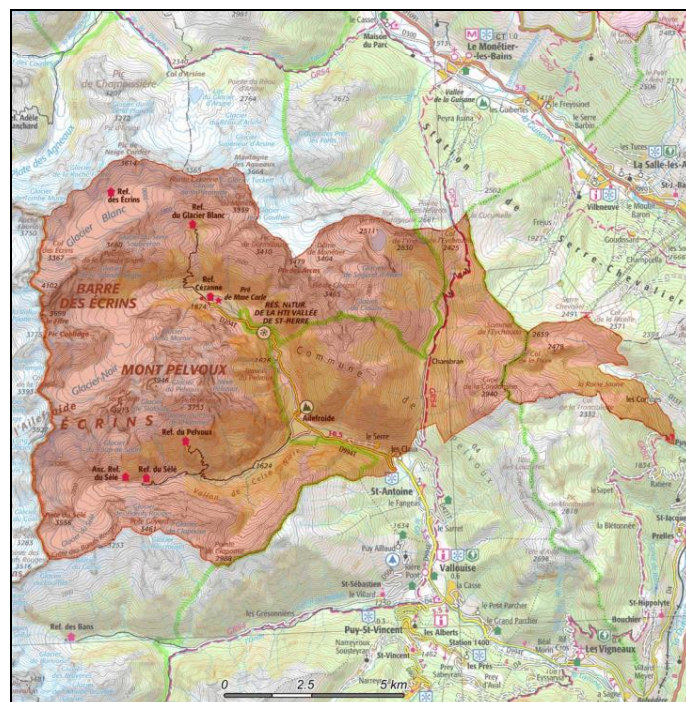
Le site classé du Massif du Pelvoux (Source : DREAL PACA)
