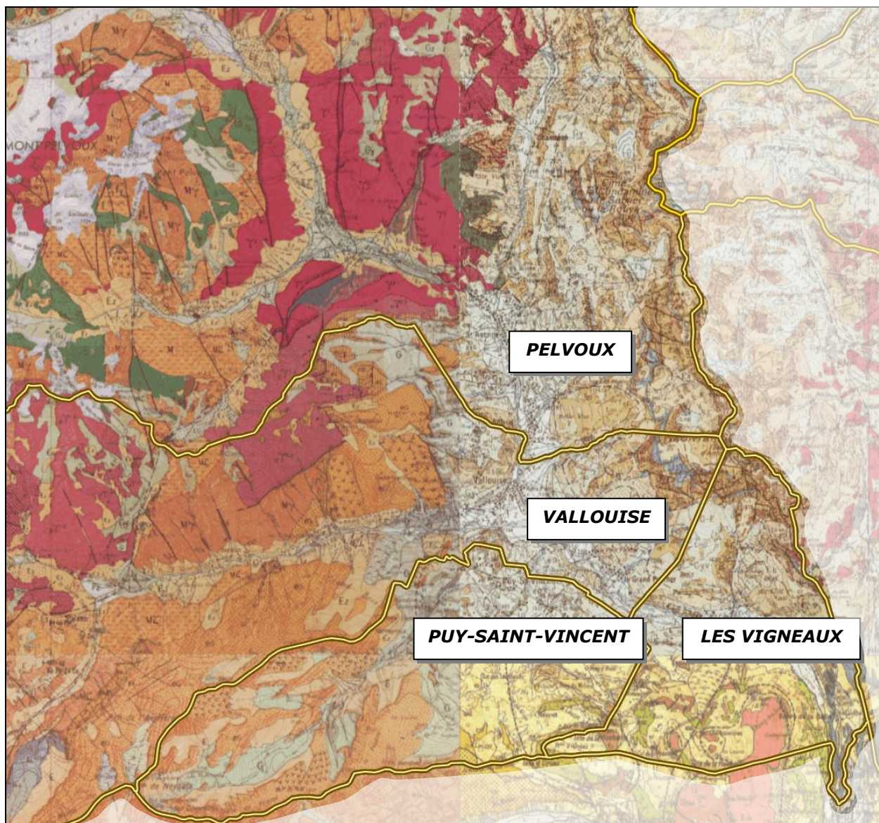
Contexte géologique de l'ensemble du territoire d'étude (Source : Géoportail)
