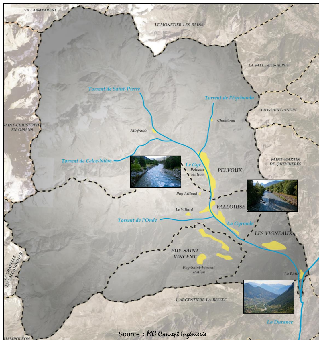
Réseau hydrographique de l'ensemble du territoire d'étude
