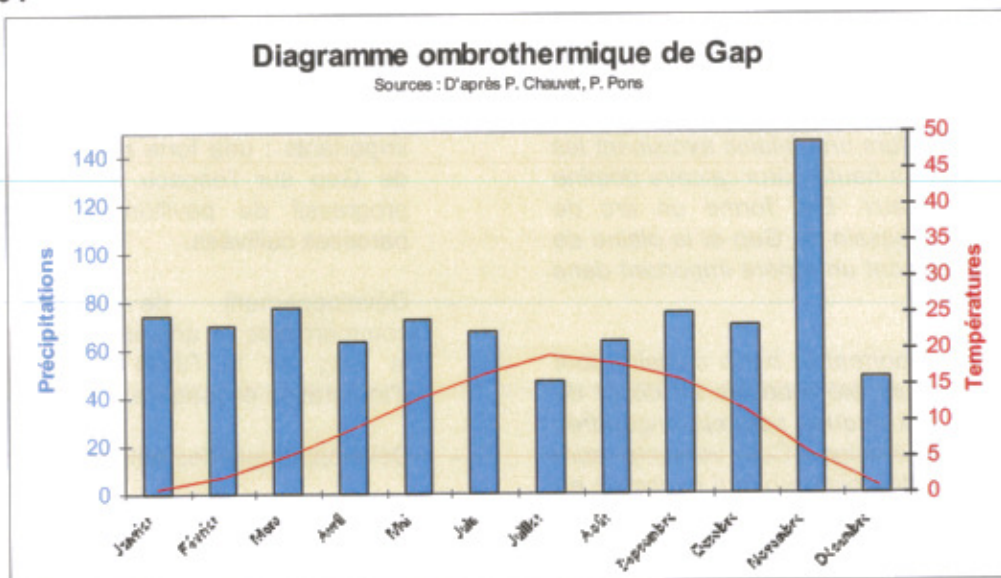
Courbe pluviométrique de Gap - Période 1961-1970 – (D'après Chauvet – Pons)
