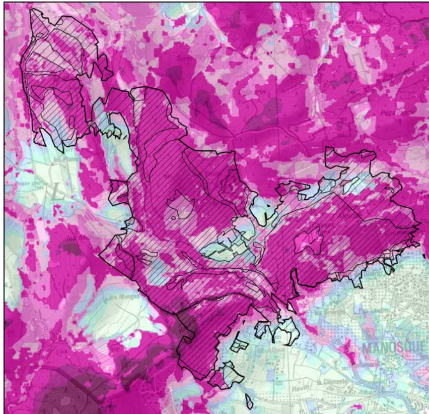
puissance de front de feu et contour de l'incendie du 07/08/2005.
