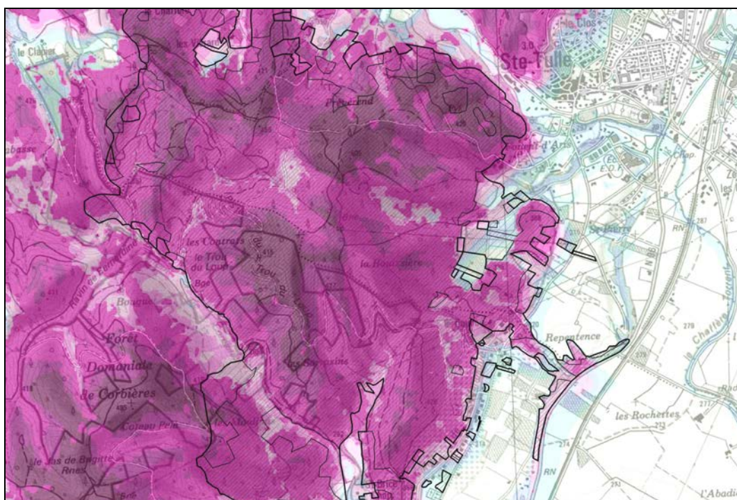
puissance de front de feu et contour de l'incendie du 24/07/2002.
