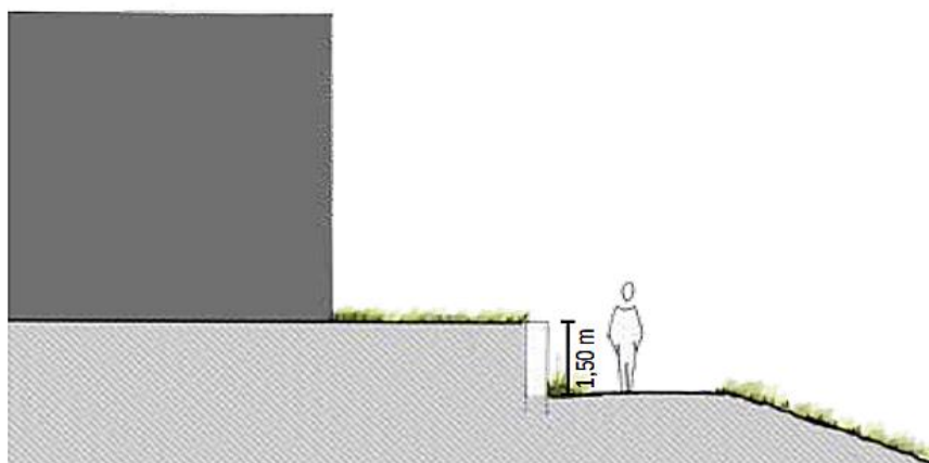
► Principe de proportion d'un soutènement
