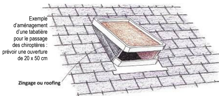
Technique de construction de la chiroptière sur tabatière
