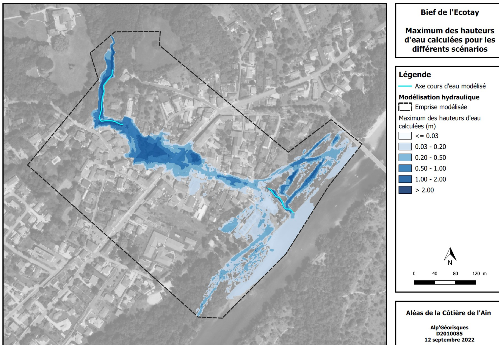
Figure IV.5: Bief de l'Ecotay – Maximum des hauteurs d'eau calculées pour les différents scénarios simulés
