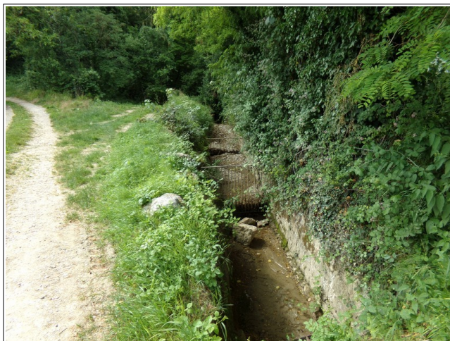
Figure II.5: ruisseau de Charmont en amont du village de Châtillon-la-Palud équipé de grilles destinées à piéger le transport solide et les embâcles. Ce dispositif est en place à l'amont immédiat d'un busage traversant le village.
