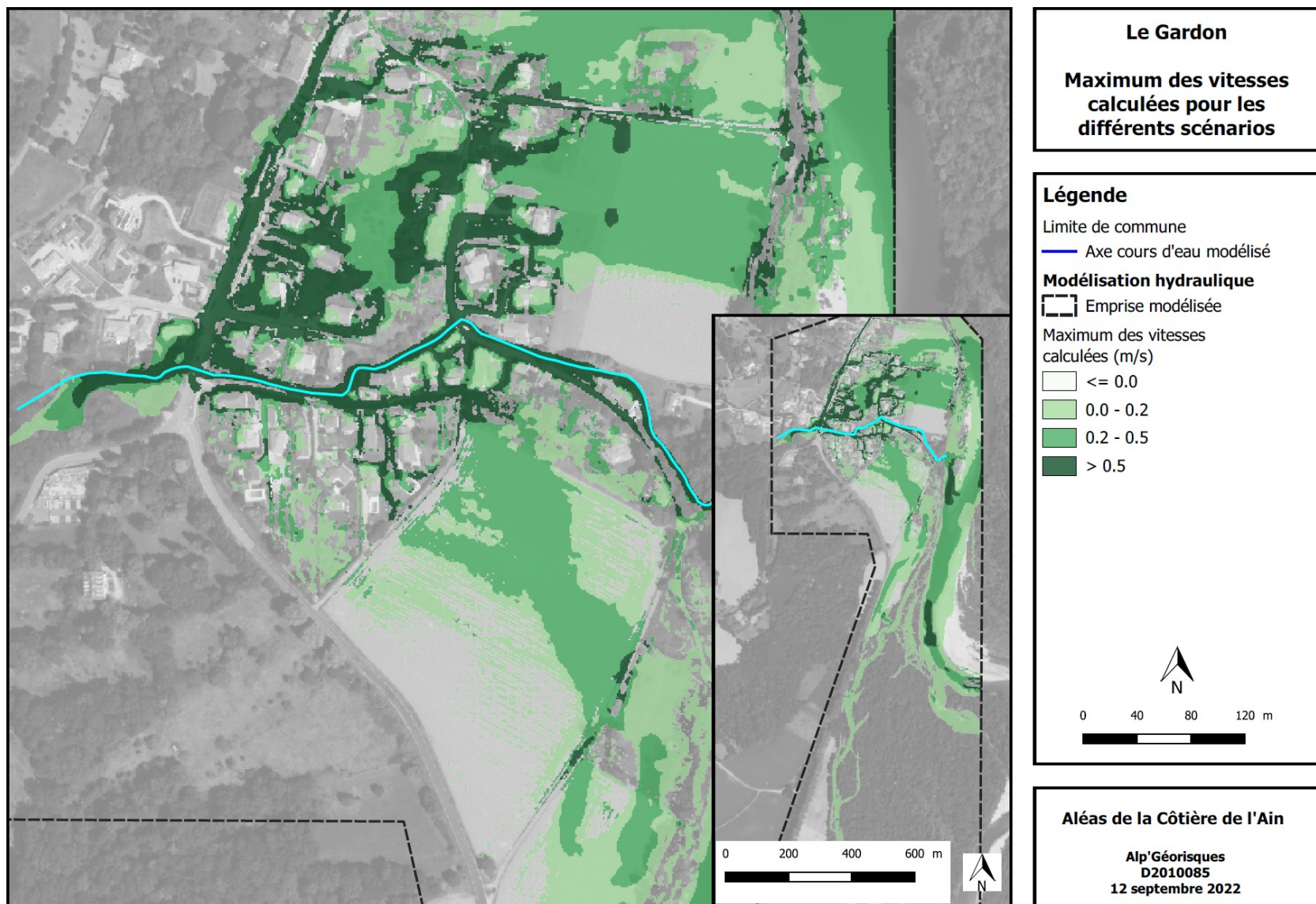
Figure IV.10: Le Gardon – Maximum des vitesses calculées pour les différents scénarios simulés
