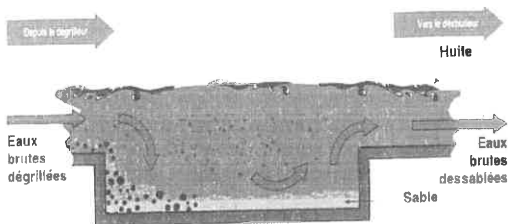
Schéma de principe du dessableur.
