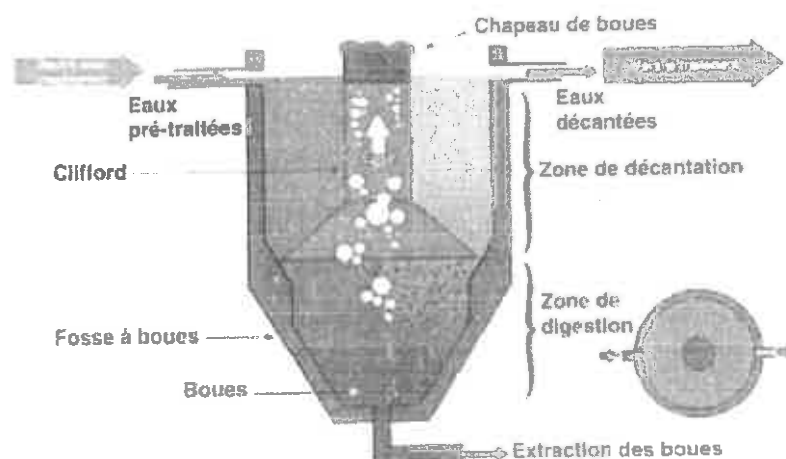
Schéma de principe du décanteur digesteur
