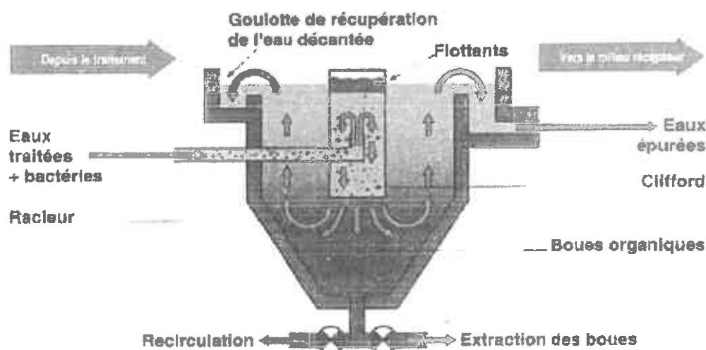
Schéma de principe du décanteur secondaire
