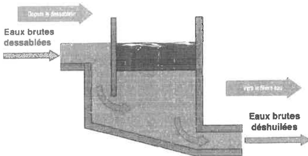
Schéma de principe du dégraisseur statique.
