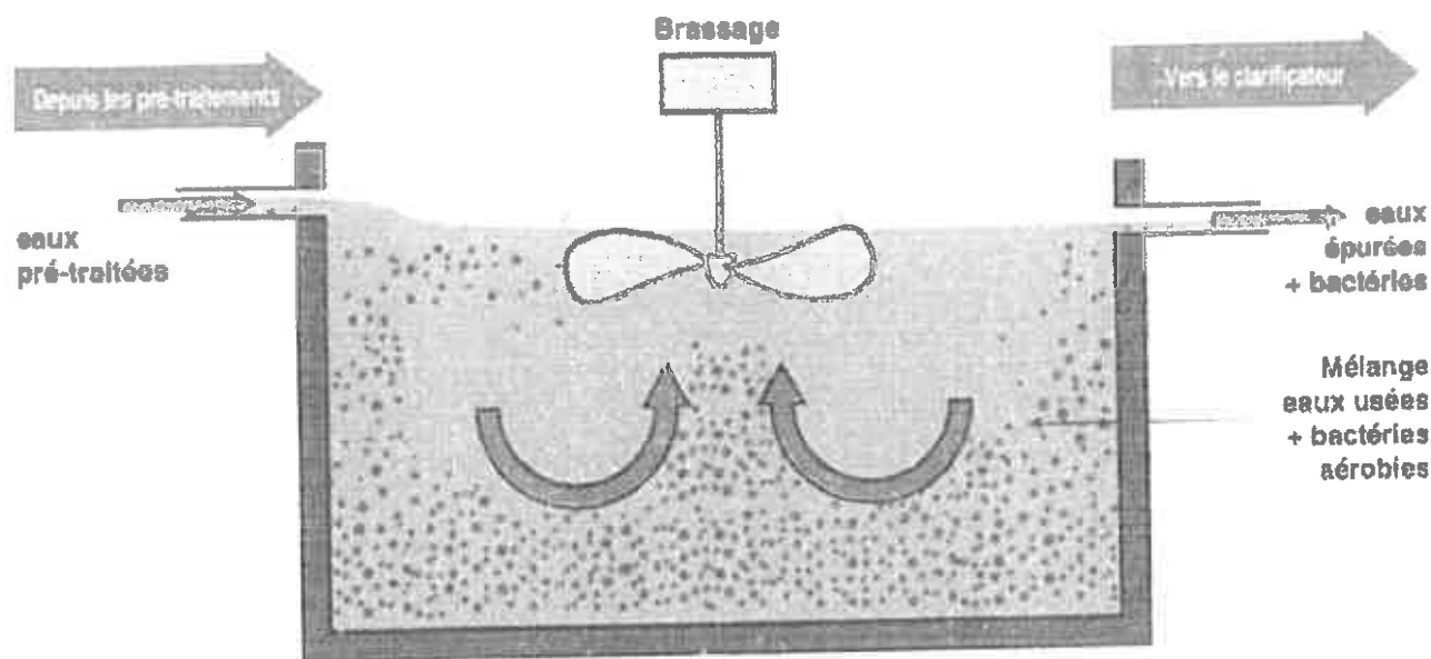
Schéma de principe du bassin d'aération.
