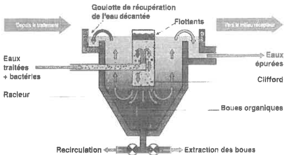
Schéma de principe du décanteur.
