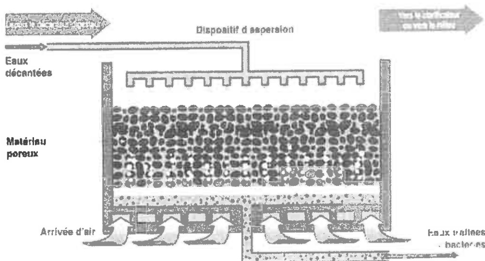
Schéma de principe du lit bactérien.
