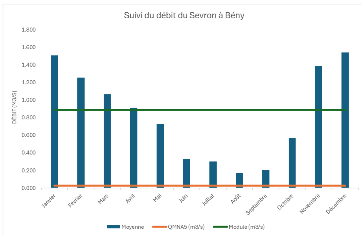
Débit mensuel moyen du Sevron à Béný depuis 2000
