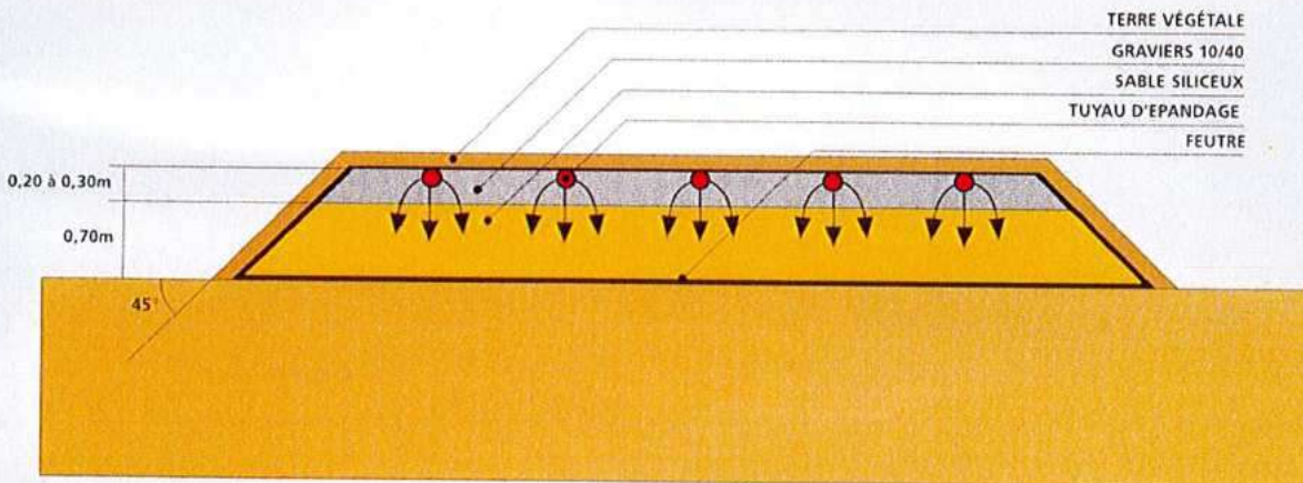
COUPE TRANSVERSALE
