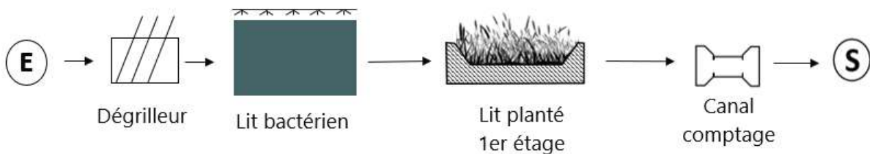
FIGURE 14 – SCHEMA DE FONCTIONNEMENT DE LA STATION D'EPURATION DE JAYAT
