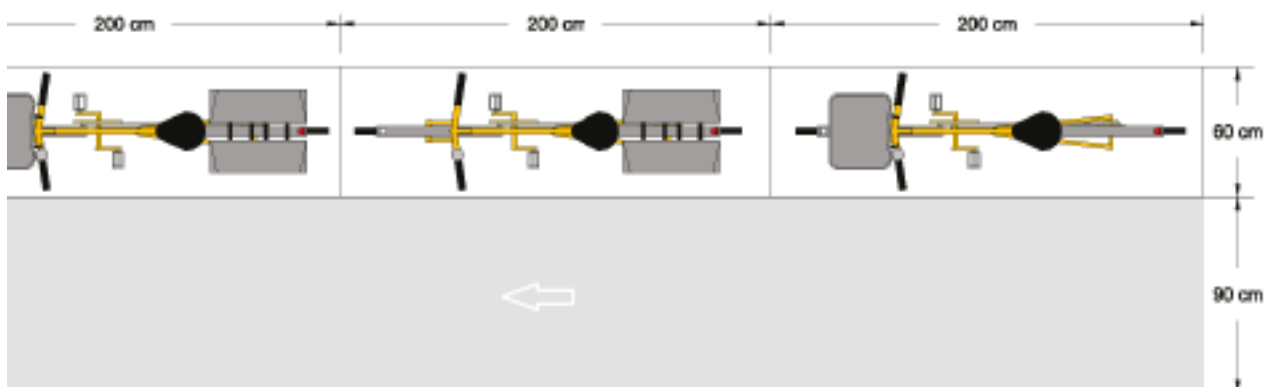
Figure 12 : Disposition longitudinale
